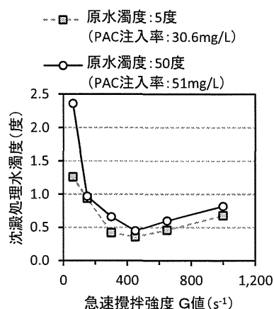
図 7-6 急速攪拌強度 (G 値) と沈澱処理水濁度の関係 [11]
