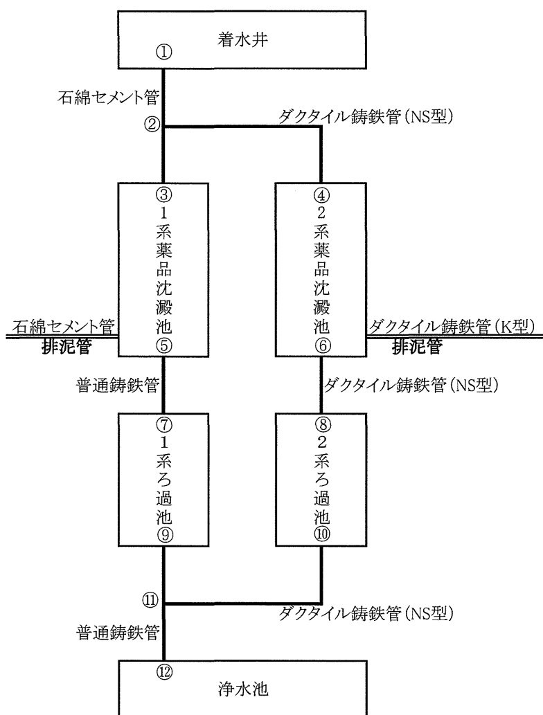
図 R5. 1 簡易耐震診断モデルの場内配管のデータ
