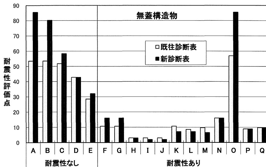
図 5 既往簡易耐震診断表と新簡易耐震診断表の診断結果の比較(無蓋構造物)
