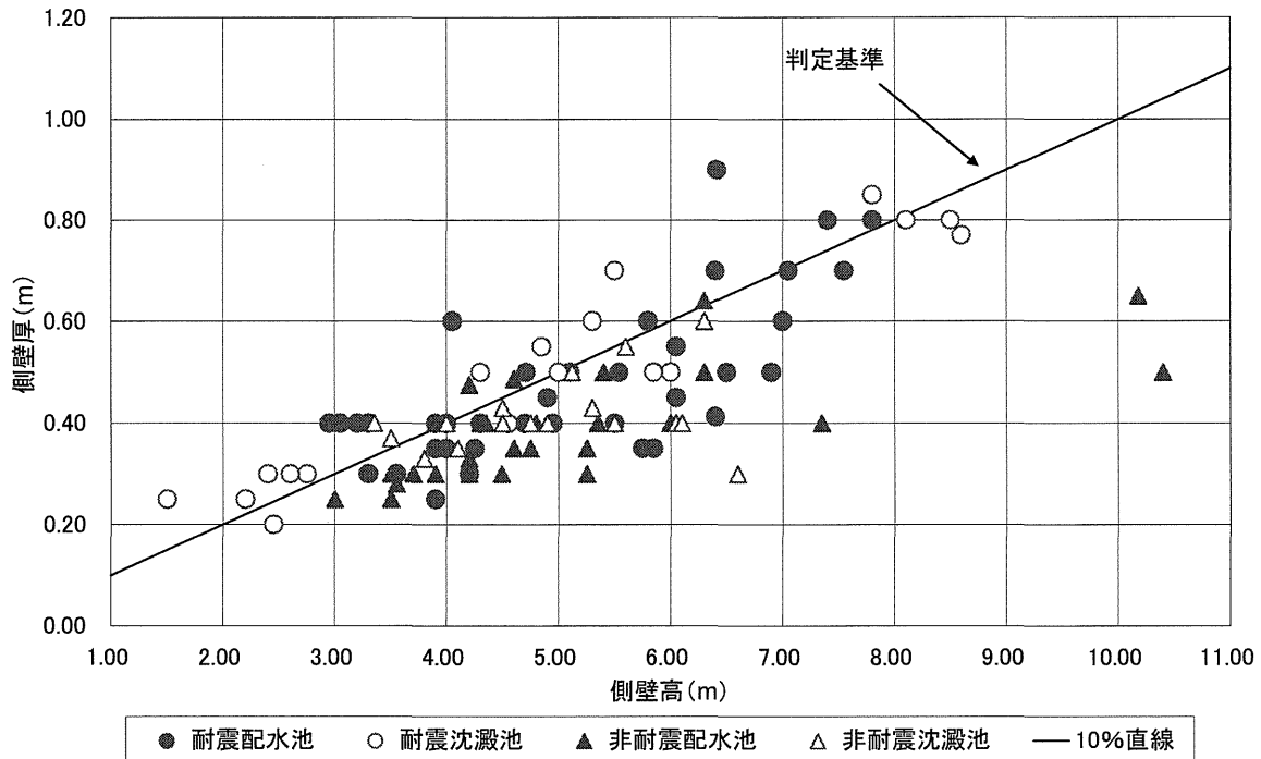
図 2 壁の高さと厚さの関係
