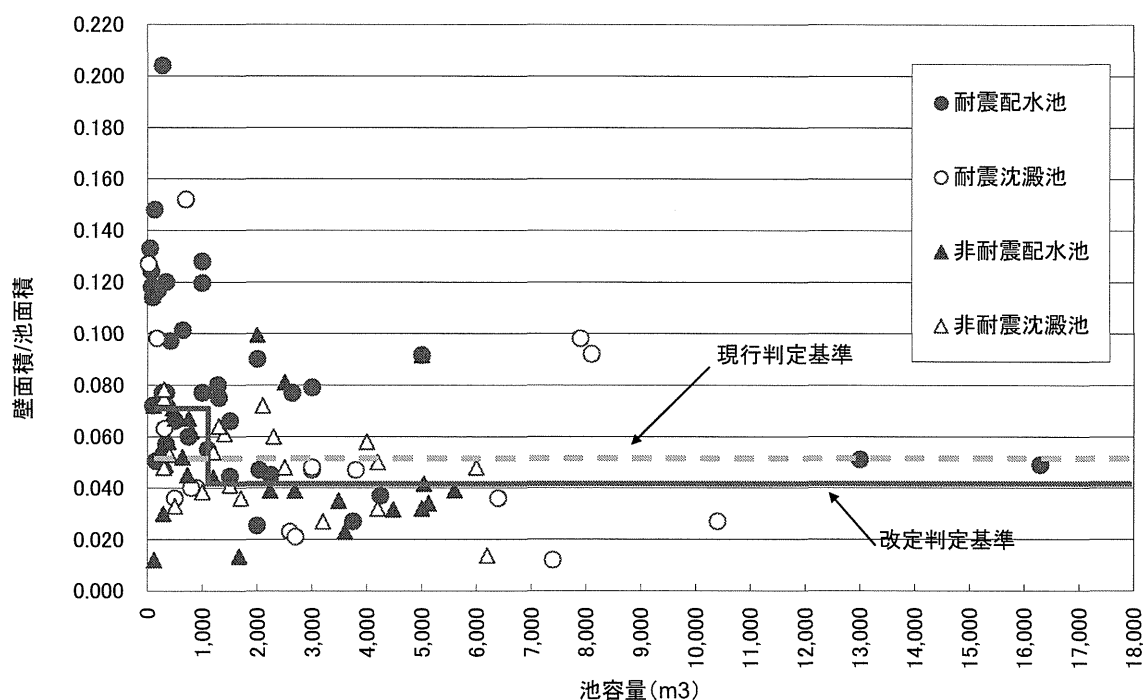
図 1 方向別壁面積/池面積比と池容量の関係
