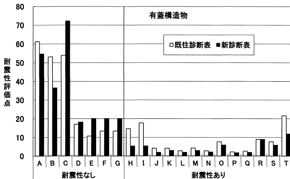
図 4 既往簡易耐震診断表と新簡易耐震診断表の診断結果の比較(有蓋構造物)
