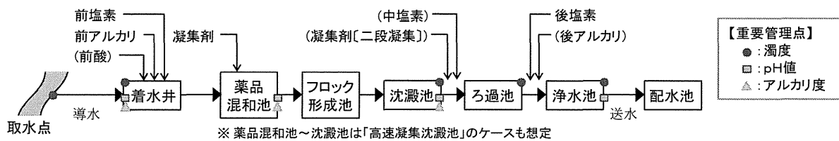
図 1 想定した浄水フロー
