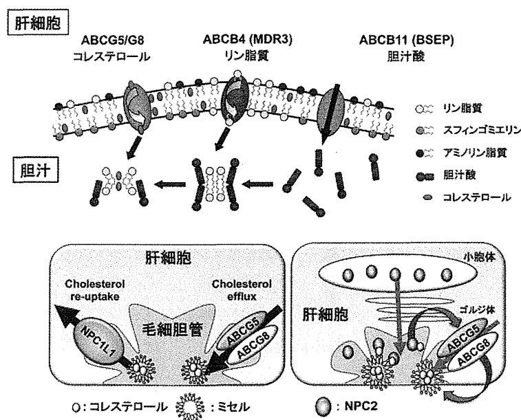
図4 コレステロール輸送担体 ABCG5/G8, NPC1L1, NPC2 の機能連関
