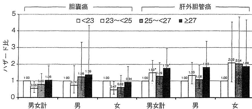
図1 肥満度と胆道癌(胆嚢癌と肝外胆管癌)(文献8より引用, 一部改変) 肥満度23未満を1とした時のリスク。
