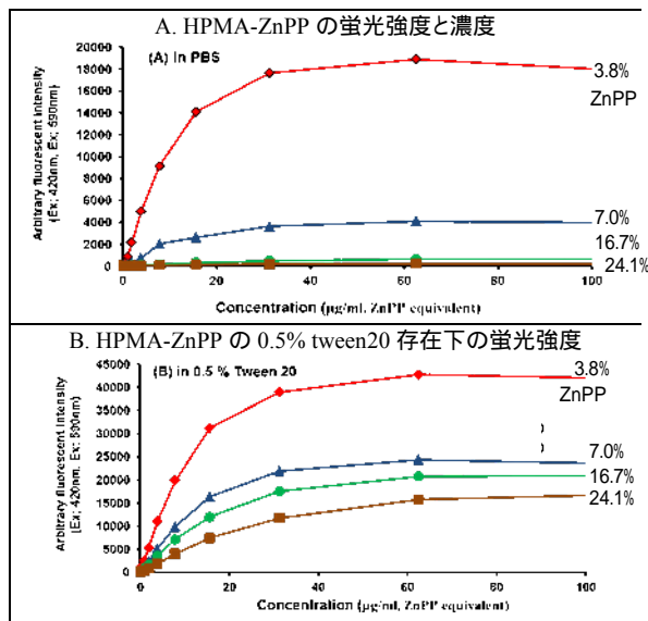
図 3. PHPMA-ZnPP の蛍光強度と一重項酸素の生成強度。ZnPP 含量の少ない HPMA-ZnPP ほど、強い蛍光を発生する。特に HPMA-ZnPP (3.8%)は強い蛍光を発生し、HPMA-ZnPP (16.7%)や HPMA-ZnPP (24.1%)と比べると、50 ~ 100 倍程度の蛍光強度を示した。Tween 20 などの界面活性剤で HPMA-ZnPP のミセル構造を壊すと、すべての HPMA-ZnPP において、蛍光の回復が認められたが、依然として ZnPP 含量の低いものにおいて高い蛍光が観察された。
