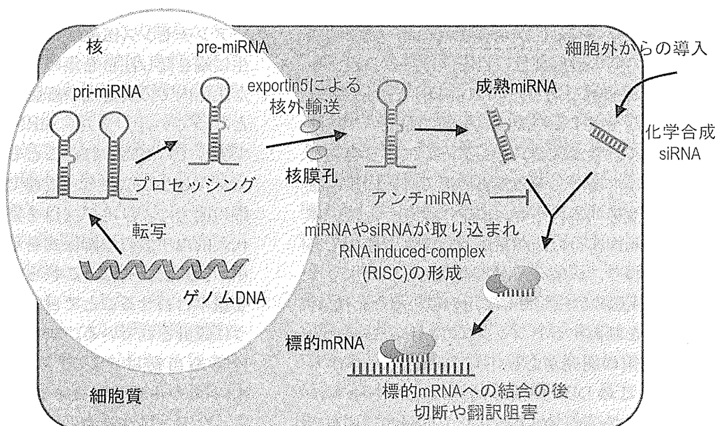
図2 内因性 miRNA と外から導入した siRNA の mRNA 阻害機構の模式図
