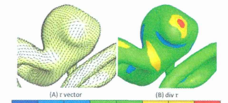
図2 数値流体解析による菲薄部位予測指標 左；流速ベクトル 右；壁面せん断応力
