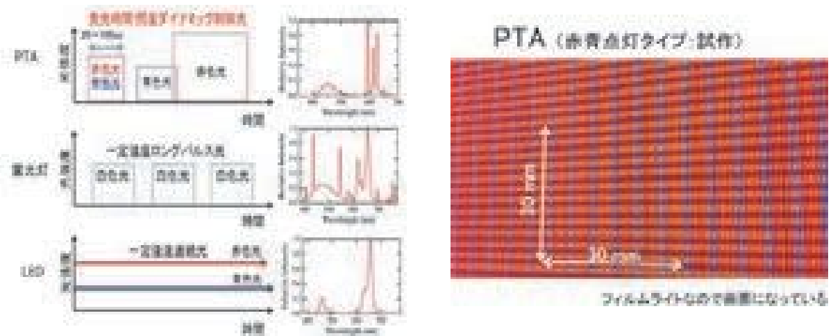
図 2 . 使用する光源の特性及びスペクトルの比較 (左) と、試作した PTA の点灯の様子 (右)
