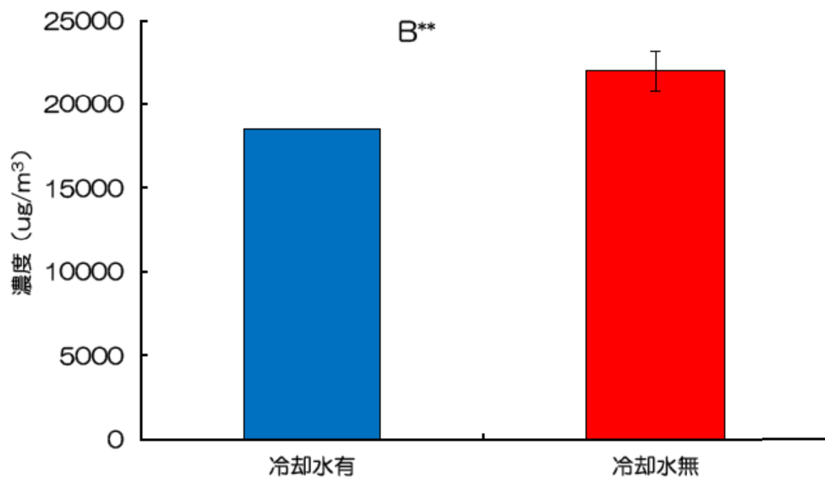
図 2-4 冷却水の有無による水銀濃度
