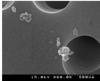
図 5.19 清掃作業時のオープン による粒子捕集例 (60000 倍)
