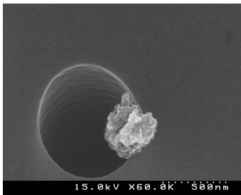
図 5.22 清掃作業時の Sioutas (E 層) による粒子捕集例 (60000 倍)
