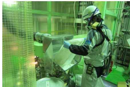
図 5.2 作業状況 2
