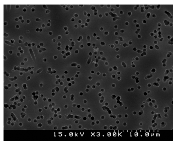
図 5.12 充填作業時の オープン による 粒子捕集例 (3000 倍)
