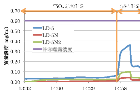
図 5.11 スポット測定における 10 分間移動平均値
