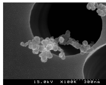
図 5.36 バックグラウンド 測定におけるオープン による粒子捕集例 (100000 倍)
