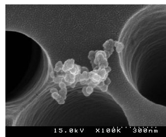
図 5.14 充填作業時の オープン による 粒子捕集例 (100000 倍)
