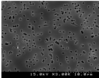
図 5.18 清掃作業時のオープン による粒子捕集例 (3000 倍)
