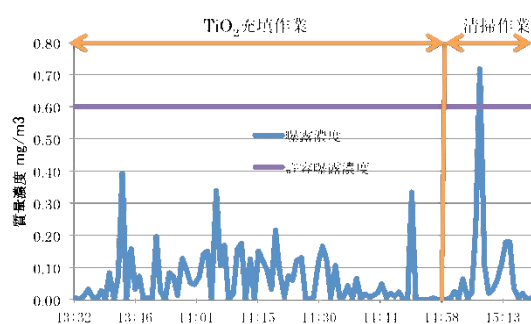
図 5.24 曝露濃度変動
