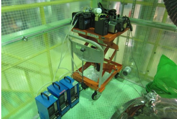
図 5.4 測定状況 1
