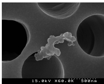
図 5.35 バックグラウンド 測定におけるオープン による粒子捕集例 (60000 倍)
