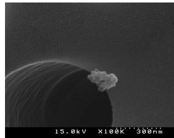
図 5.31 清掃作業時の LD-6N による呼吸器付近の粒子捕集例 (100000 倍)
