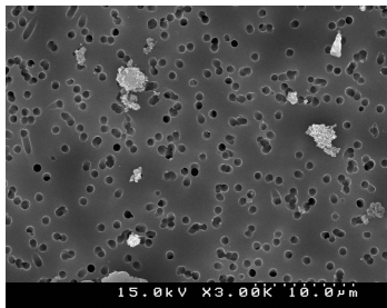
図 5.26 充填作業時の LD-6N による呼吸器付近の粒子捕集例 (3000 倍)
