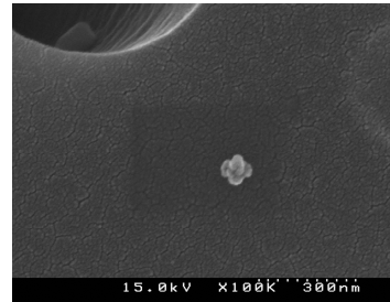
図 5.20 清掃作業時のオープン による粒子捕集例 (100000 倍)
