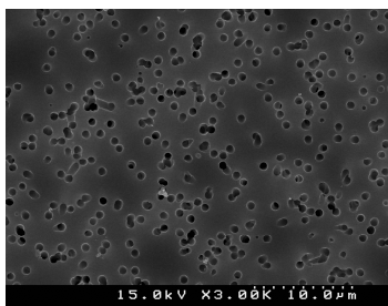
図 5.34 バックグラウンド 測定におけるオープン による粒子捕集例 (3000 倍)
