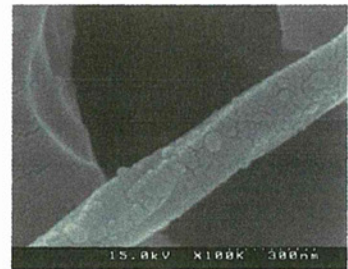
図 1.79 MWCNT, 1.0×10 -8 wt%の FE-SEM 観察結果(100000 倍)
