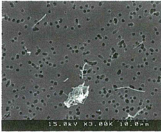
図 1.72 MWCNT, 1.0×10 -6 wt%の FE-SEM 観察結果(3000 倍)
