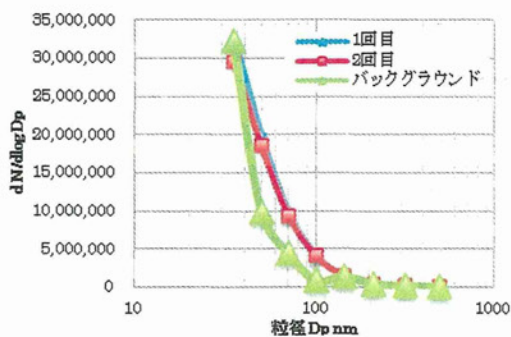
図 1.41 50nmTiO 2 ,1.0×10 -8 wt% の粒度分布
