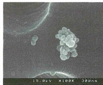
図 1.40 50nmTiO 2 , 1.0×10 -6 wt%の FE-SEM 観察結果(×100000)
