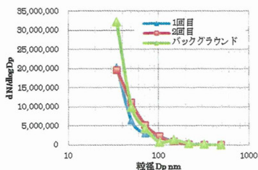
図 1.70 MWCNT, 1.0 \times 10^{-6}\text{wt}\% の粒度分布
