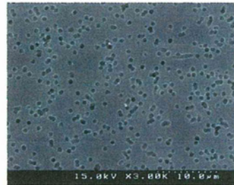
図 1.106 銀ナノ粒子の 1.0 \times 10^{-8} wt% の FE-SEM 観察結果(30000倍)
