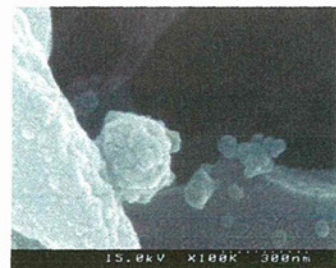
図 1.89 フラーレン 1.0×10 -4 wt%の FE-SEM 観察結果(100000倍)
