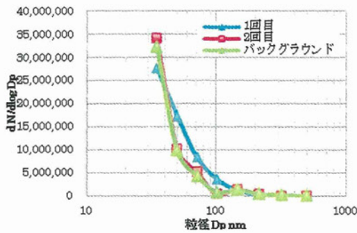
図 1.75 MWCNT, 1.0×10 -8 wt%の粒度分布
