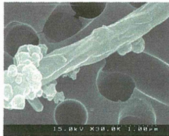
図 1.78 MWCNT, 1.0×10 -8 wt%の FE-SEM 観察結果(30000 倍)
