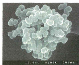
図 1.45 50nmTiO 2 , 1.0×10 -8 wt%の FE-SEM 観察結果(×100000)
