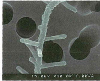
図 1.73 MWCNT, 1.0×10 -6 wt%の FE-SEM 観察結果(30000 倍)
