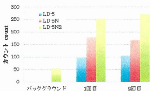
図 1.95 LD-5、LD-5N、LD-5N2 による計測値（フラレーン、 1.0 \times 10^{-4} wt%）
