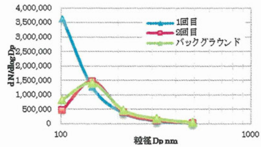
図 1.76 MWCNT, 1.0×10 -8 wt%の 粒度分布 (100~500nm)
