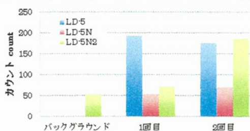
図 1.80 LD-5、LD-5N、LD-5N2 による計測値(MWCNT, 1.0 \times 10^{-6}\text{wt}\% )
