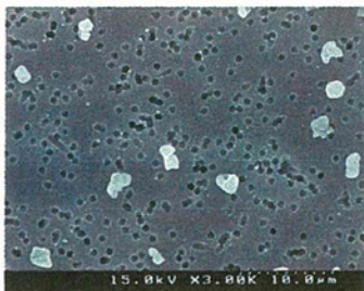
図 1.87 フラーレン 1.0×10 -4 wt%の FE-SEM 観察結果(3000倍)
