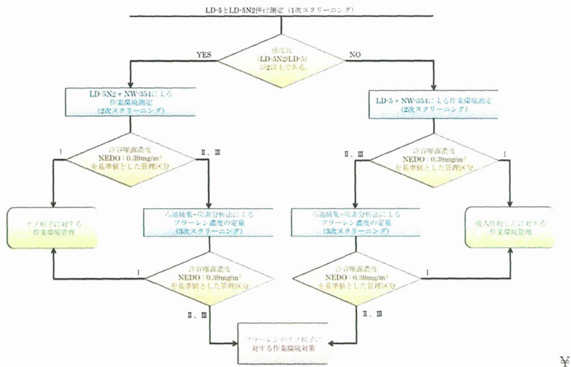
図 1.97 フラーレン取扱い作業現場における作業環境管理フロー
