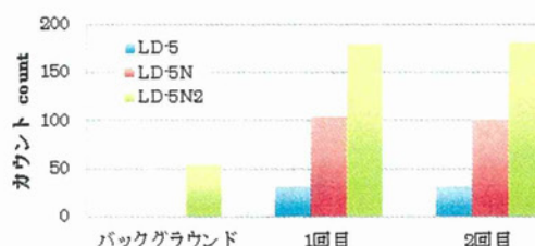
図 1.96 LD-5、LD-5N、LD-5N2 による計測値（フラレーン、 1.0 \times 10^{-6} wt%）
