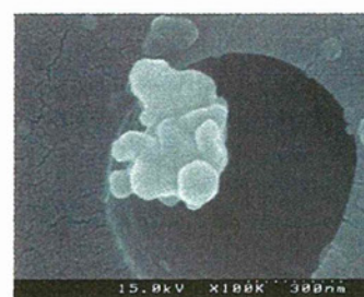
図 1.102 銀ナノ粒子の 1.0 \times 10^{-6}\text{wt}\% FE-SEM 観察結果(100000倍)
