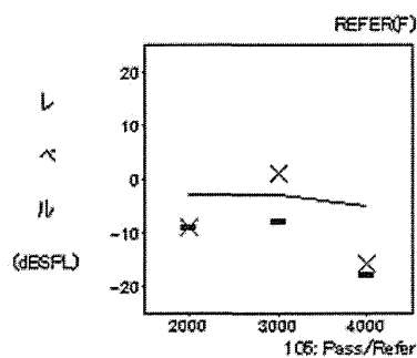
Referの例
