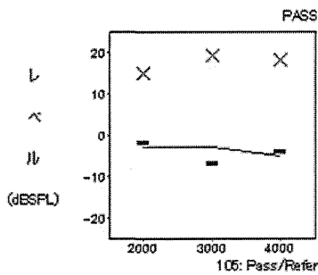
Passの例
