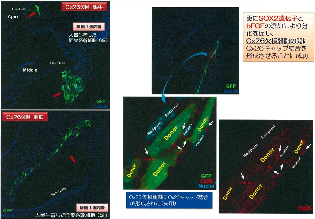
図 新規開発したコネクシン 26 欠損マウスへの CCR2 遺伝子導入間葉系幹細胞 (MSC-CCR2) の導入。移植した MSC-CCR2 は内耳組織を生着し細胞間に欠損していた Cx26 が含まれるギャップ結合プラークを構築させることに成功した。
