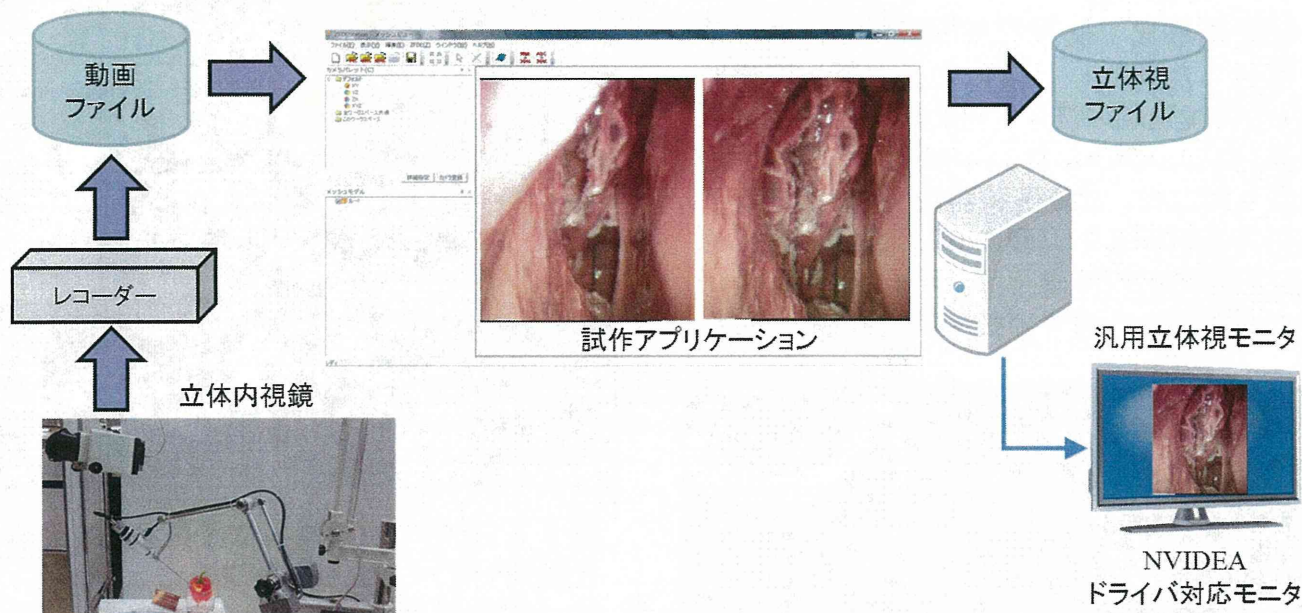
図 18 立体視表示システム（立体視モニタへの出力）
