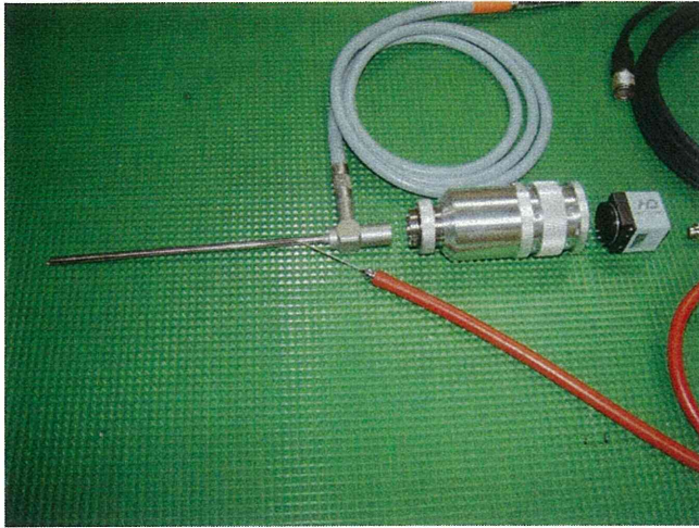
図 1 2 新型カメラアタッチメントおよび CMOS ハイデフィニションカメラ、光源ファイバーの全体像
