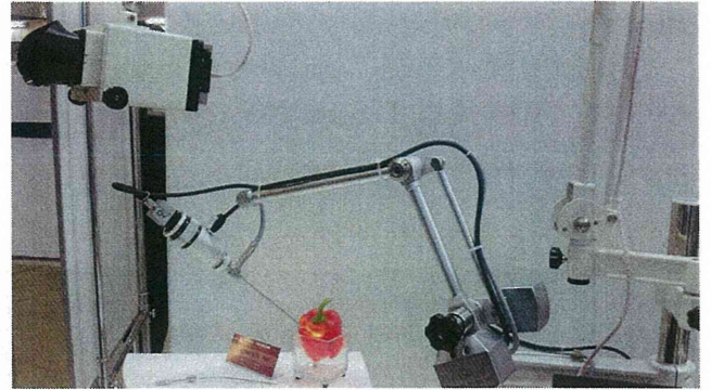
図 1 4 立体内視鏡システム本体に接続された鏡筒
