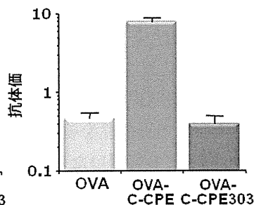
図3 Claudin binder を利用した粘膜ワクチン
