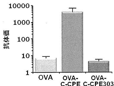
図3 Claudin binder を利用した粘膜ワクチン
