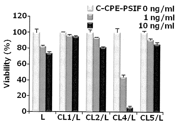
図2 Claudin-4 指向性分子
