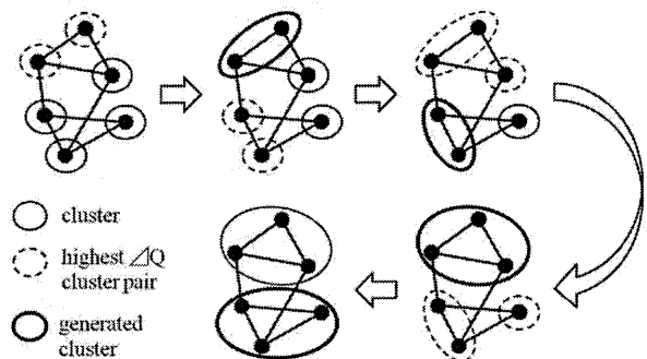
図2 単語の連結
