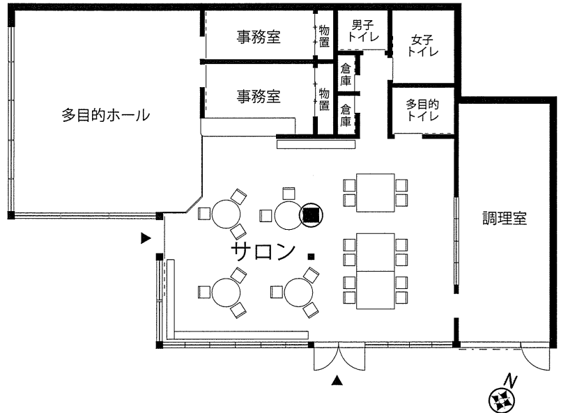
1 F PLAN 1/200
