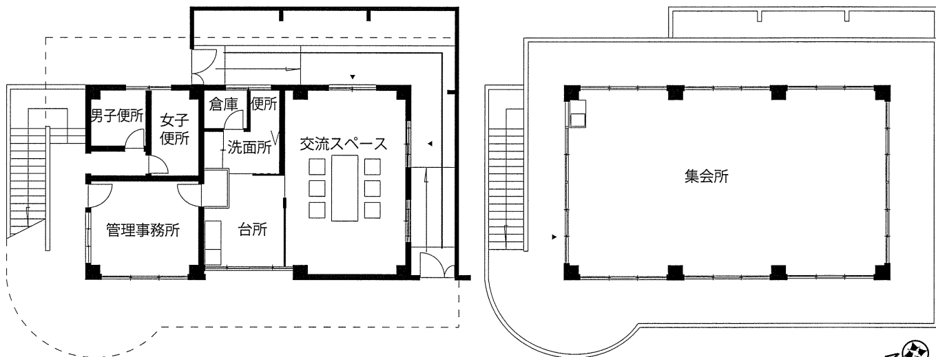
1 F PLAN 1/200
