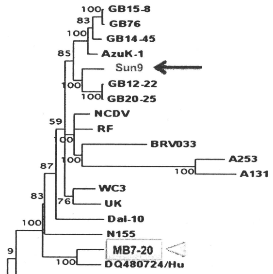
図 1. 牛から分離されたロタウイルスの VP1 及び VP2 遺伝子の遺伝学的関係
