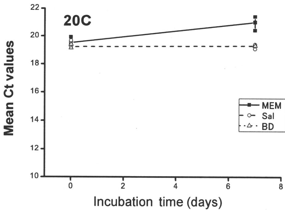
図2 ウイルスゲノムの検出
