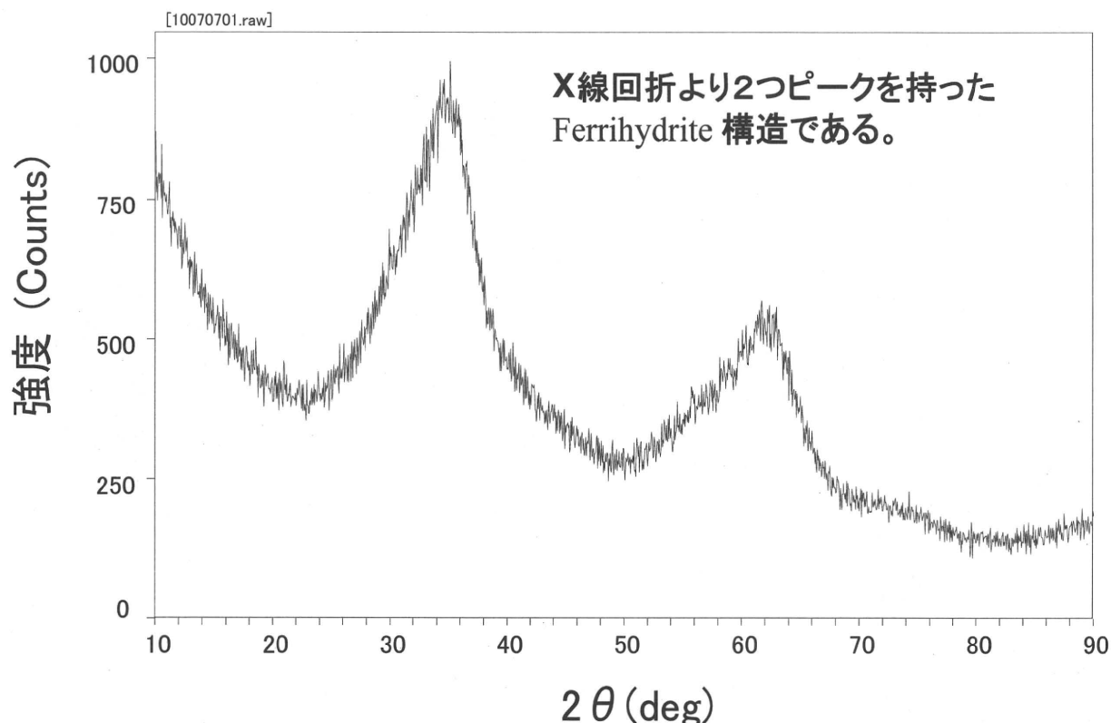
図2 非晶質鉄 (aFe) の強度分析. Ferrihydrite構造であることが認められた。
