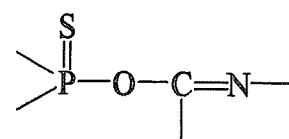
図1 共通構造
