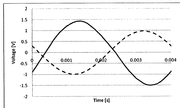
図 1 - 1 8 : 両面テープ（事務用）、250Hz
