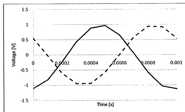
図 1 - 2 0 : 両面テープ（事務用）、1000Hz
