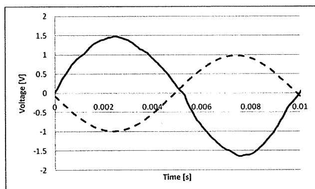
図 1 - 1 7 : 両面テープ（事務用）、100Hz
