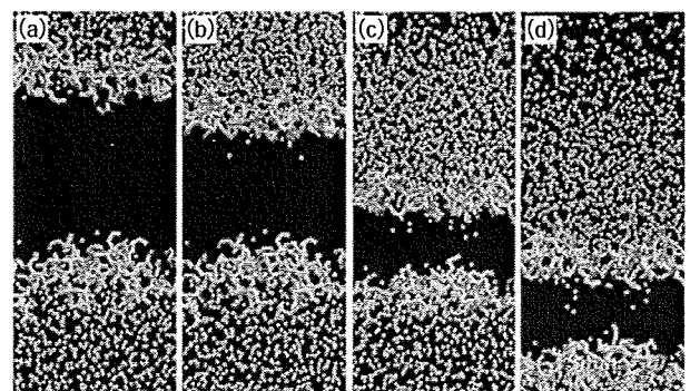
図5 衝撃波インパルス作用後の脂質二重膜の構造変化 衝撃波インパルスの作用を受けた脂質二重膜の変形を分子動力学シミュレーションで解析する。水分子を青色で表記し、アシル鎖は水分子の動きを理解しやすいように色付けしていない。(a) 平衡状態、(b) 0.15ps 後には疎水基に水分子が移動し始める、(c) 0.30ps、(d) 0.45ps。平衡状態にあっても、水分子は疎水基に存在する 3) 。
