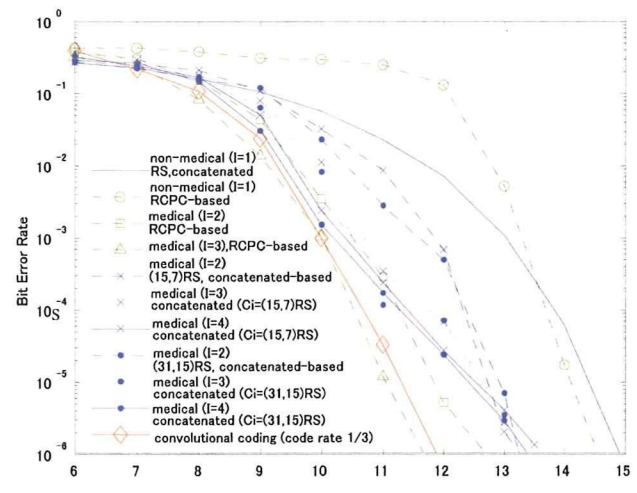
図 2 ビット誤り率
