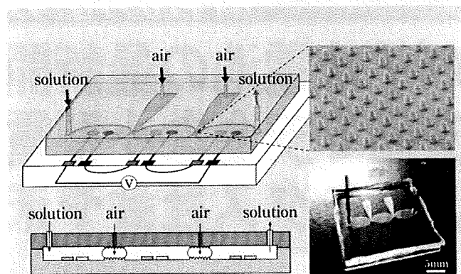
図2 MEMSバイオ電池 超撥水エアバルブによる自動スタッキング
