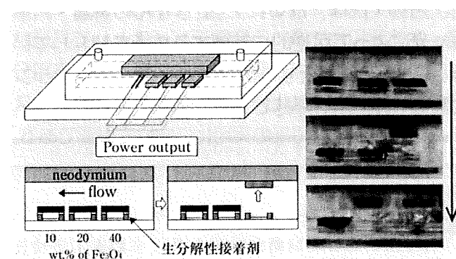
図3 MEMSバイオ電池 時差式発電システムによる長寿命化の試み
