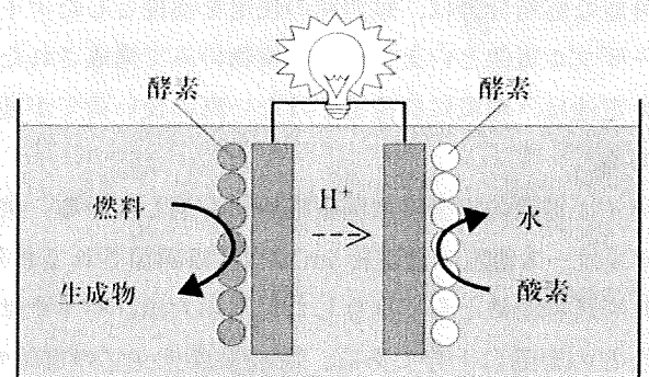
図1 バイオ電池の構造
