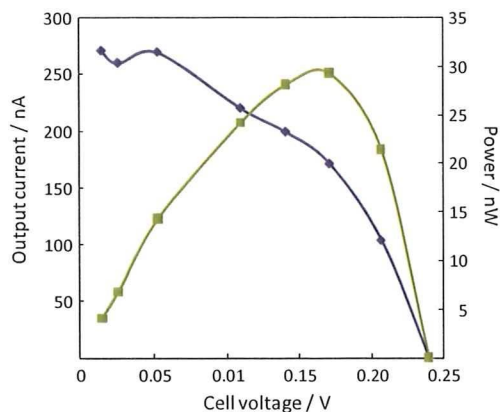
図 C-3-3 バイオ燃料電池出力（血清中測定）
