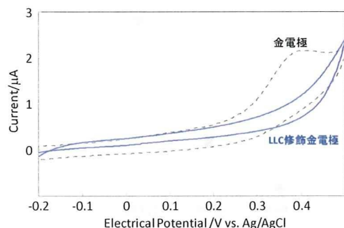
図 C-3-1 血液中でのサイクリックボルタモグラム
