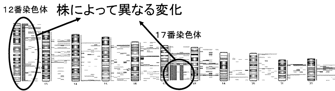
図5. MRC-5 およびヒト iPS 細胞 5 株のアレイ CGH 解析
