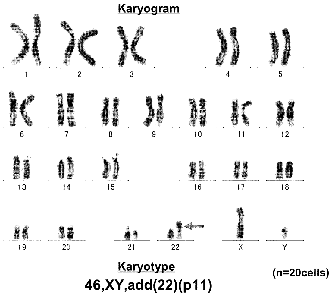
図2. ヒト iPS 細胞 (JCRB1329:Squeaky) の G-band 法による染色体解析
