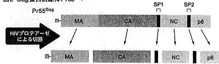
Gag 蛋白前駆体 Pr55Gag はマトリックス (MA)、キャプシド (CA)、ヌクレオキャプシド (NC) と p6 ドメインの4つの主領域と、CA-NC 間、NC-p6 間にある SP1、SP2 からなる。
