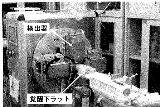
(a) 開発した小動物用 SPECT 装置
