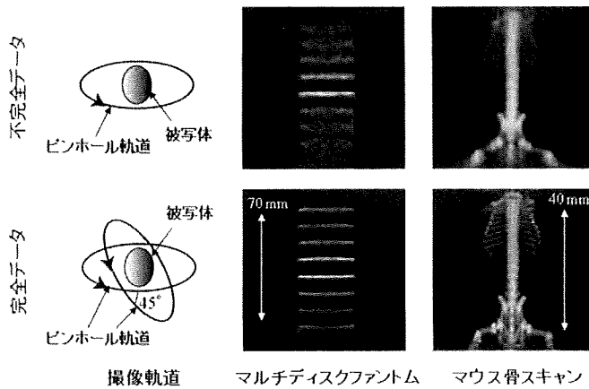
図 2 従来の単一円軌道による不完全データ (上) と 2 軸収集軌道による完全データ (下) から得られた再構成画像
