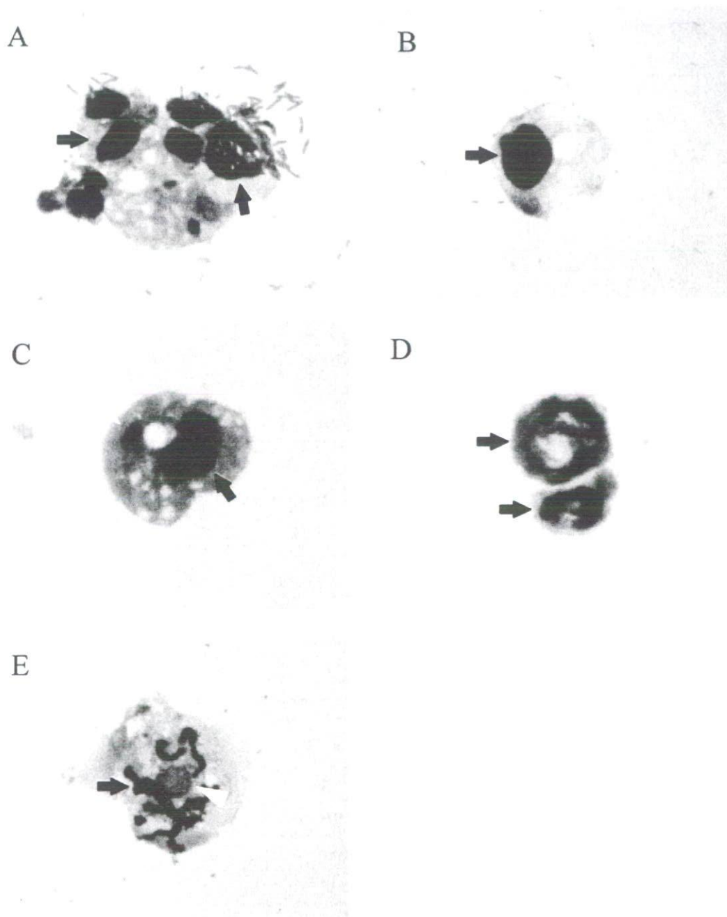
図-1、 L. londiniensis の感染アメーバ細胞内増殖 (感染 2 日後)
