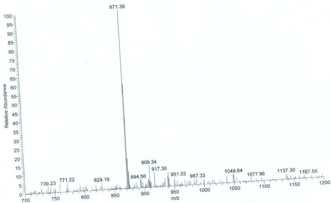
図 8 - b PTX3精製品のMSスペクトル (陰イオンモード)
