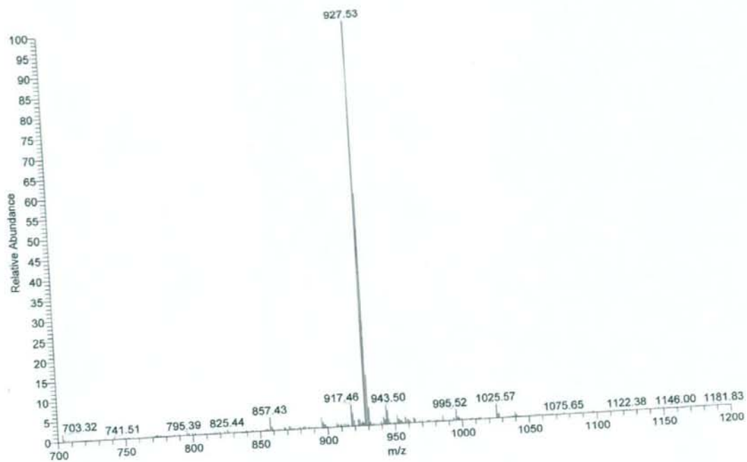
図8-c PTX3精製品のMSスペクトル (陽イオンモード)
