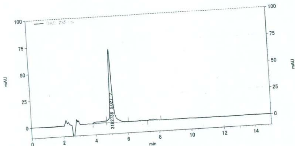
図 8 - a PTX3精製品のHPLC測定結果
