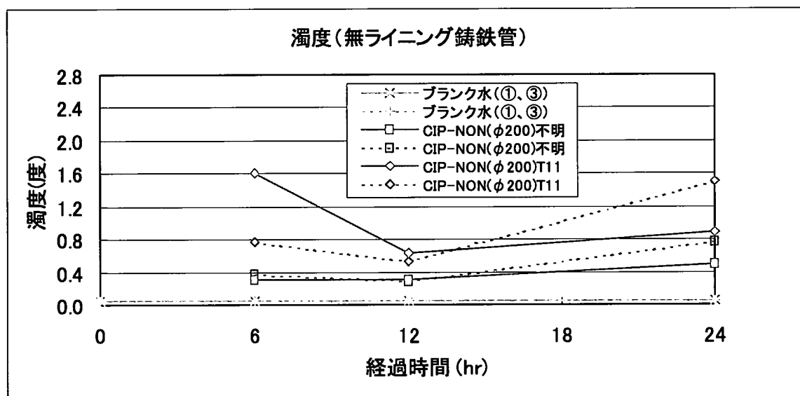
図 3.5.32 濁度 無ライニング鑄鉄管
