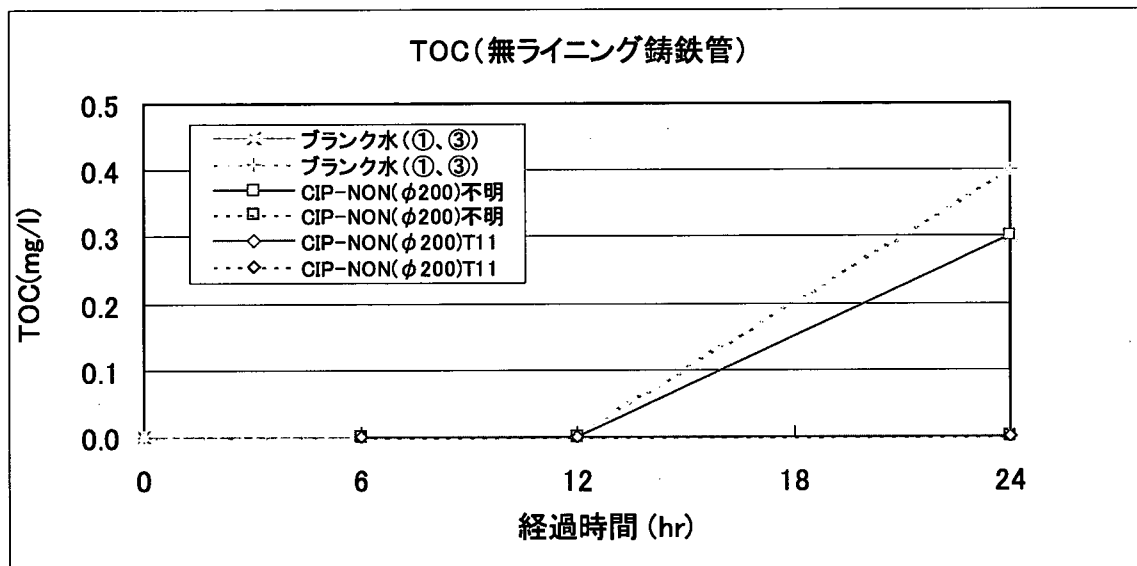
図 3.5.36 TOC 無ライニング鉄管
