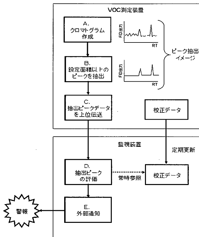
図 41 ガスクロマトグラフ VOC 測定装置による臭気原因物質警報システム案
