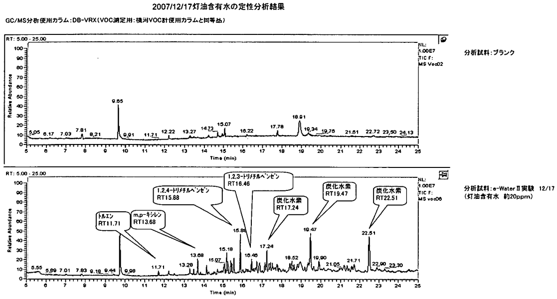
図 22 A 事業者による灯油含有水の GC/MS 測定結果 (1)
