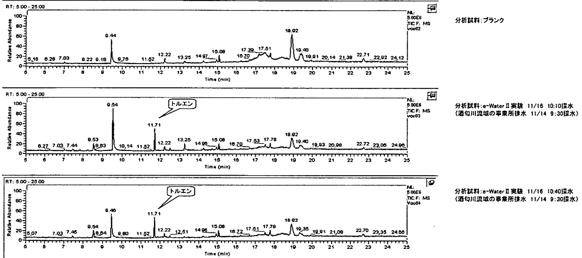
図 25 A 事業体によるトルエン含有水の GC/MS 測定結果
