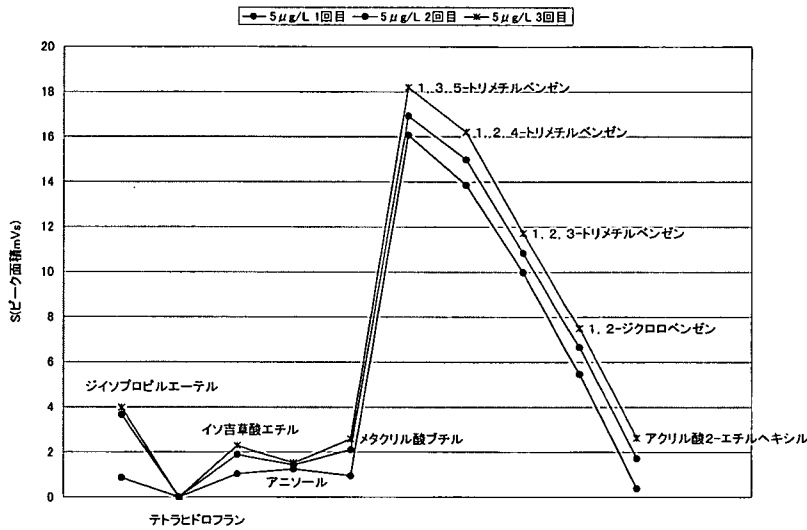
図 10 委員会選定 10 物質 5 \mu g/L 希釈時の VOC 測定装置のピーク面積
