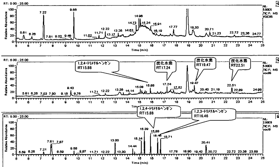
図 20 A 事業体による軽油含有水のGC/MS測定結果
