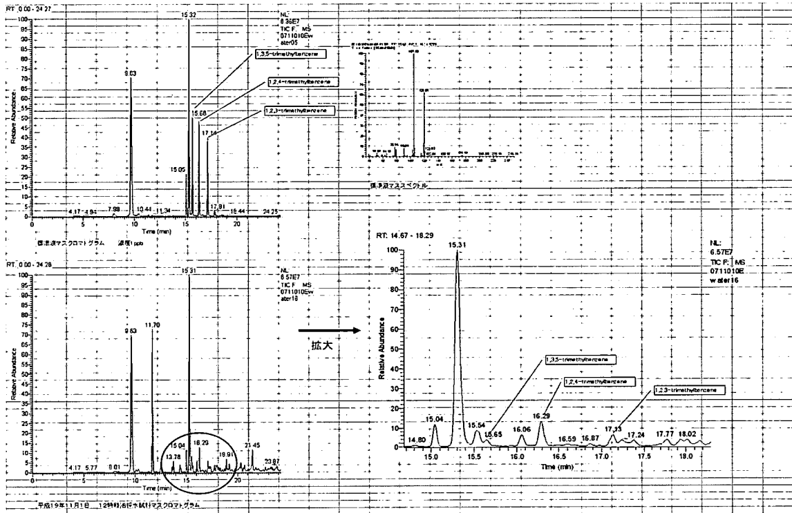
図 21 B 事業体による軽油含有水のGC/MS測定結果
