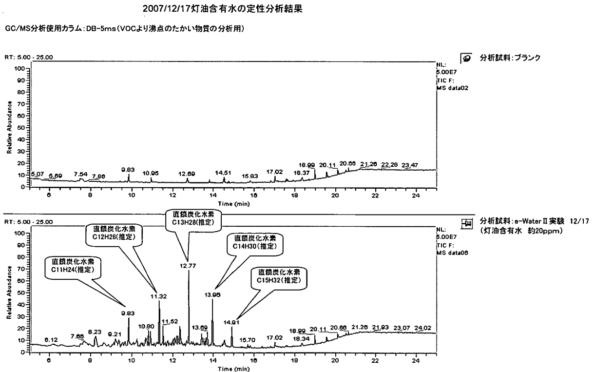
図 23 A 事業者による灯油含有水の GC/MS 測定結果 (2)
