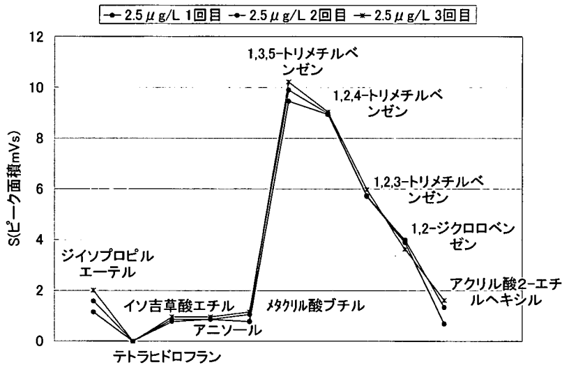
図 11 委員会選定 10 物質 2.5 \mu g/L 希釈時の VOC 測定装置のピーク面積
