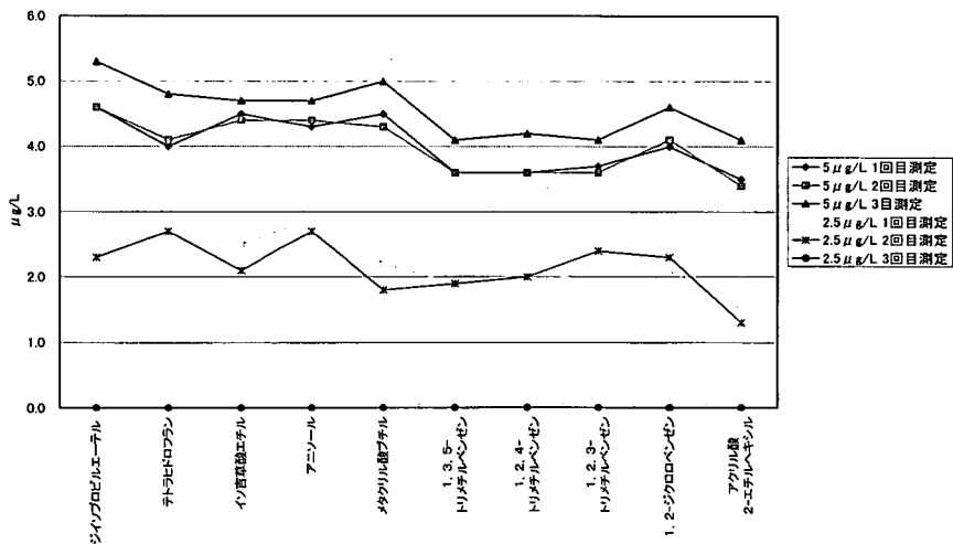
図 12 委員会選定 10 物質 5 \mu g/L および 2.5 \mu g/L 希釈時の GC/MS 測定値
