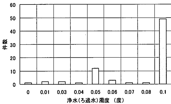
図 3-5-1 浄水 (ろ過水) 濁度管理基準値
