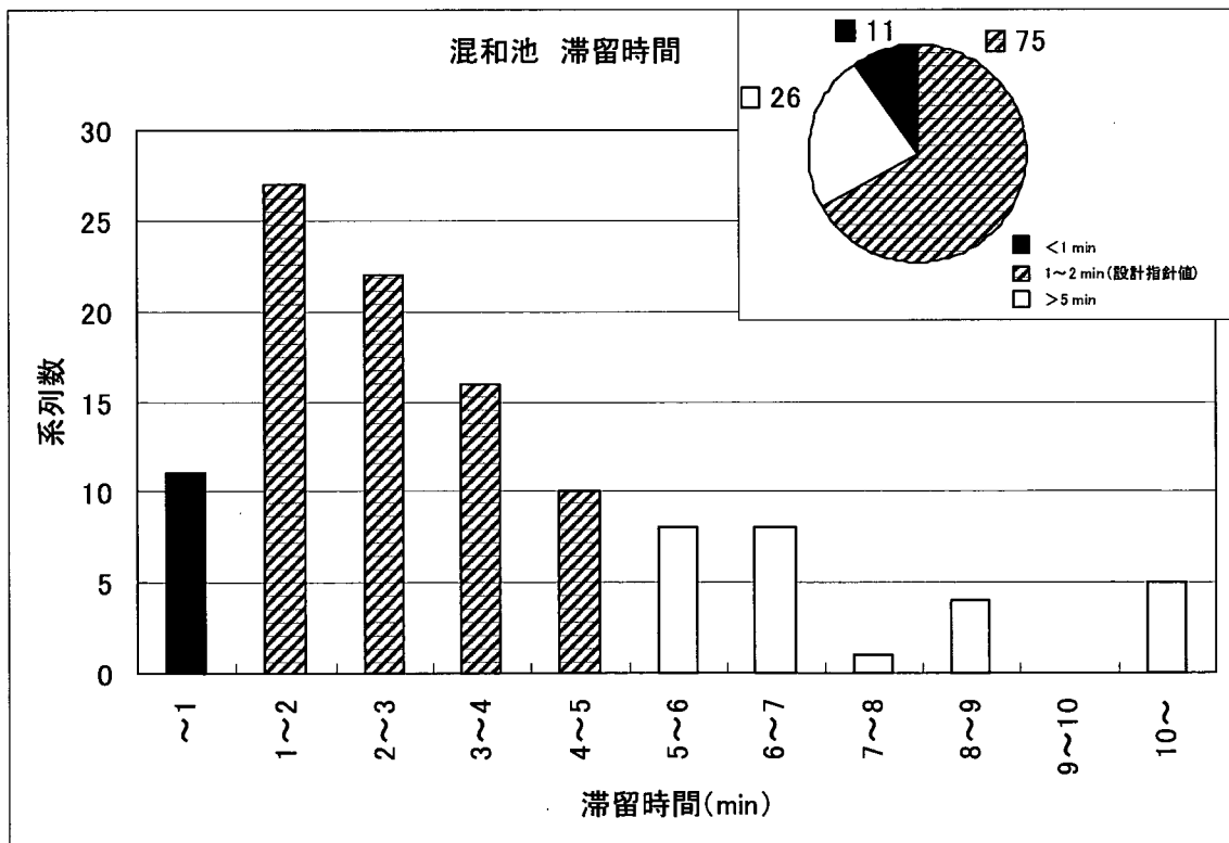
図 3-5-20 設計指針値と実績値の比較 (混和池 滞留時間)
