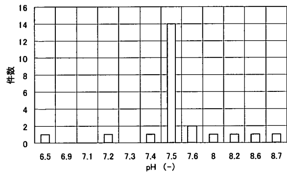
図 3-5-4 pH 上限管理基準値
