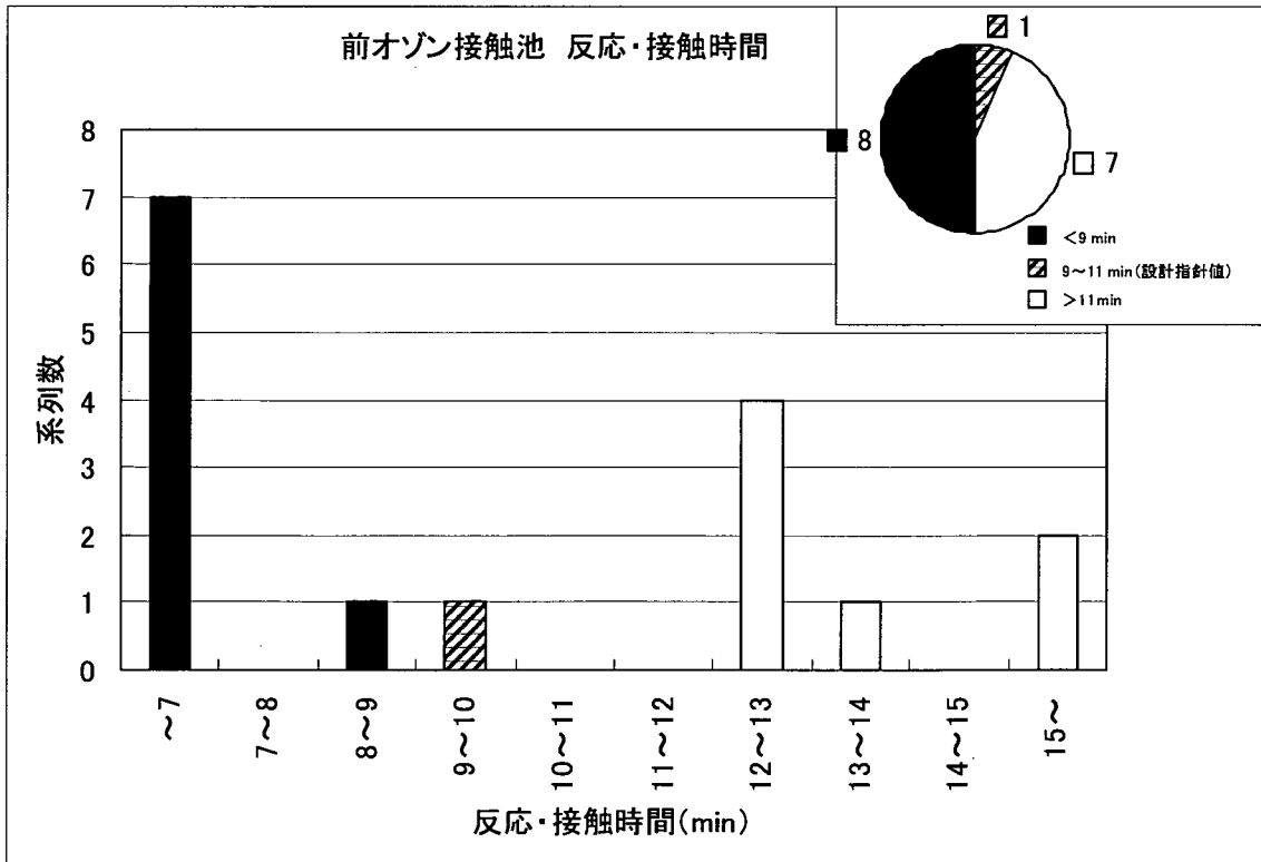
図 3-5-14 設計指針値と実績値の比較（前オゾン接触池 反応・接触時間）
