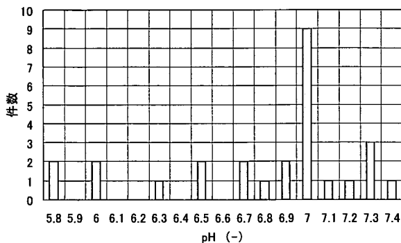
図 3-5-3 pH 下限管理基準値
