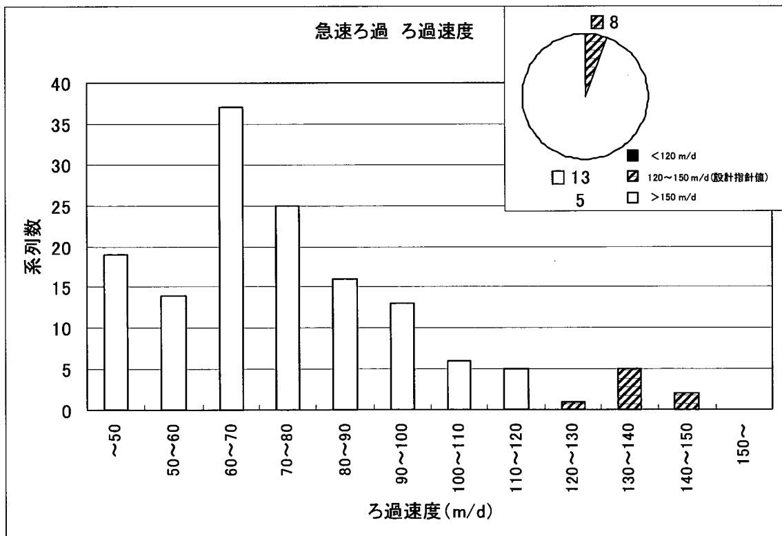
図 3-5-16 設計指針値と実績値の比較 (急速ろ過 ろ過速度)
