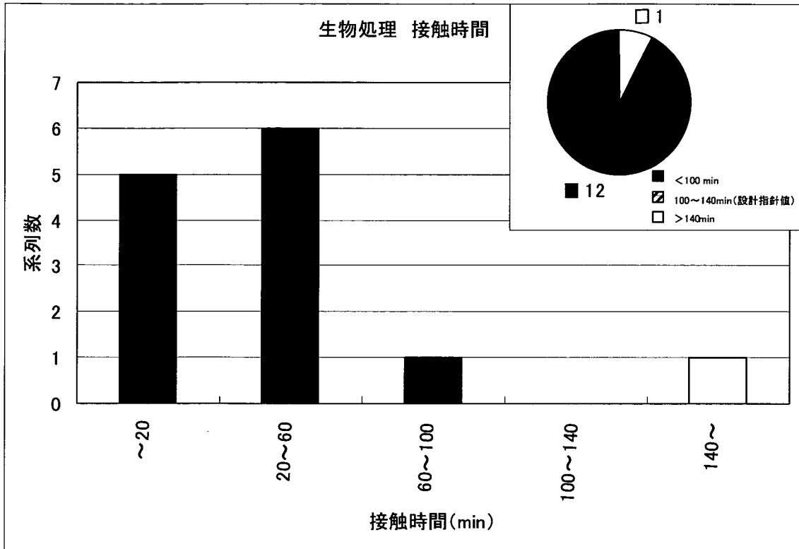
図 3-5-13 設計指針値と実績値の比較（生物処理 接触時間）
