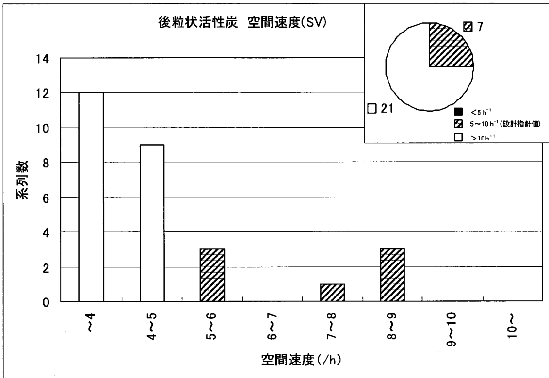
図 3-5-19 設計指針値と実績値の比較 (後粒状活性炭 空間速度)
