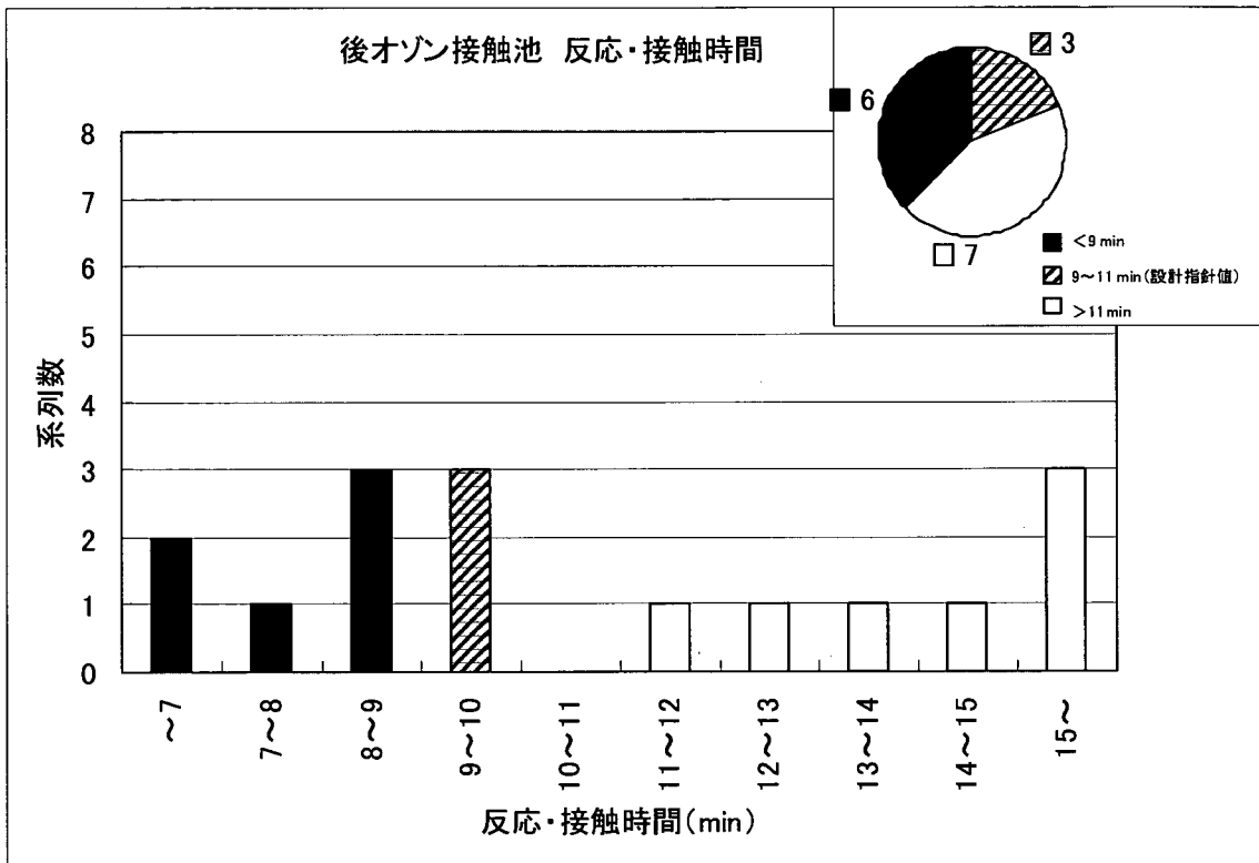
図 3-5-15 設計指針値と実績値の比較 (後オゾン接触池 反応・接触時間) ※後オゾン：急速ろ過の後にオゾン処理があるもの。
