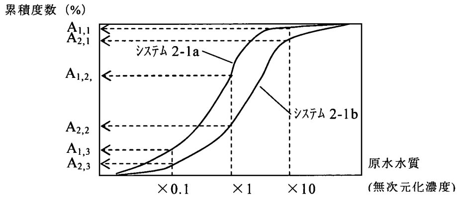
図 5-25 累積分布図
