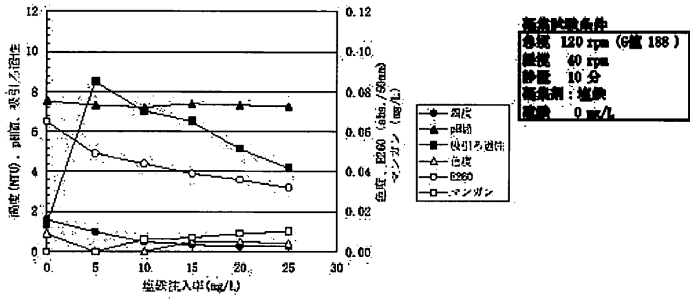
図-F-1 塩鉄注入率と処理水質の関係(凝集沈降)
