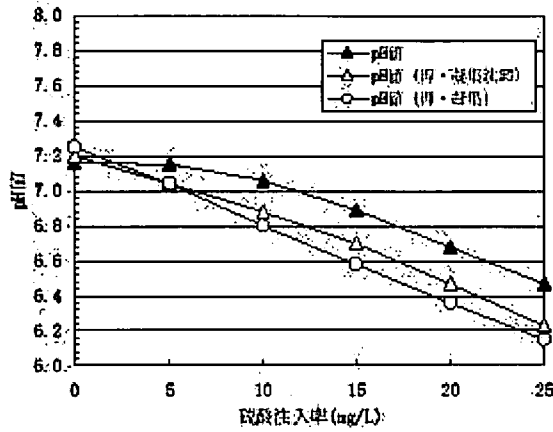
図-F-2-2 硫酸注入率とpH値の関係(塩鉄-凝集沈澱)
