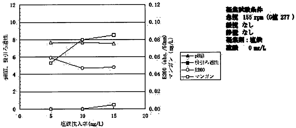
図-F-1 塩鉄注入率と処理水質の関係(高濃のみ)
