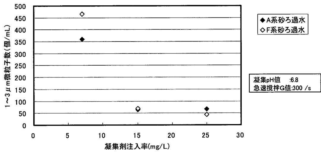
図 13 凝集剤注入率と砂ろ過水 1~3 \mu m 微粒子数の関係 [平均値]
