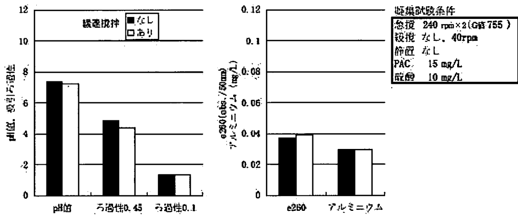
図-A-8 緩撹撹拌の有無と処理水質の関係 (静置なし)
