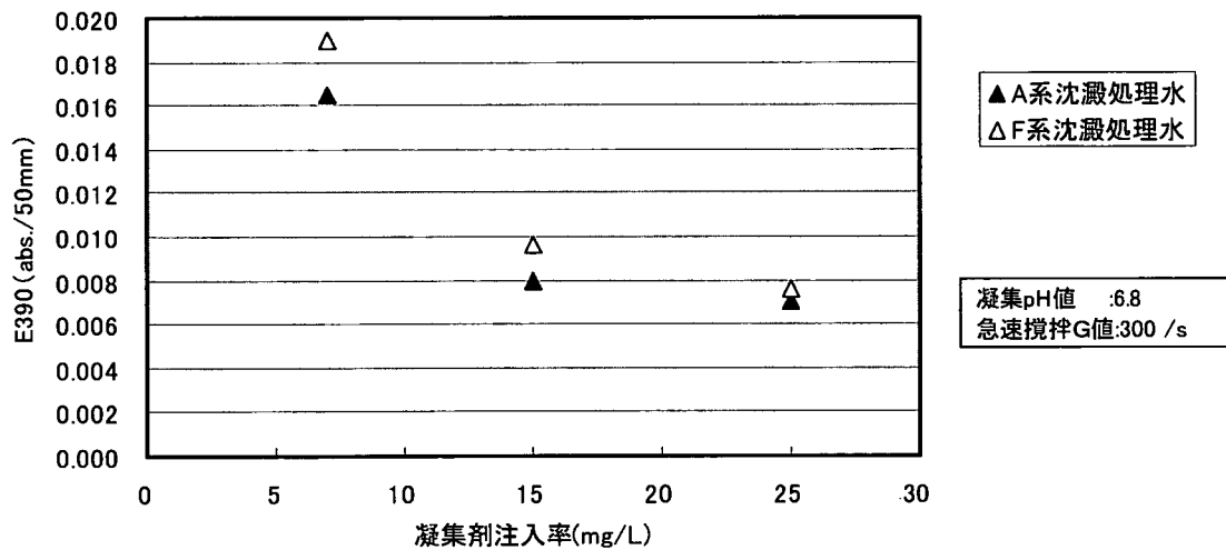
図9 凝集剤注入率とE390の関係[平均値]
