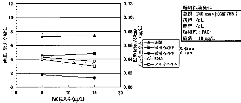
図-A-7 試験条件におけるPAC注入率と処理水質の関係 (濁集のみ)
