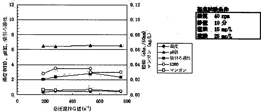
図-F-3 急速攪拌G値と処理水質の関係(凝集沈降)
