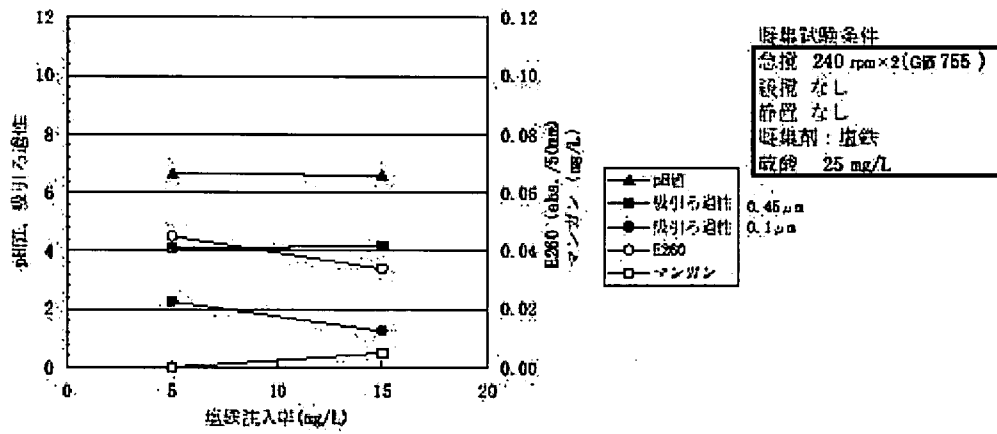
図-F-7 最適条件における塩鉄注入率と処理水質の関係(薬集のみ)
