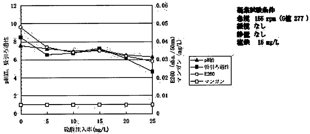
図-F-2 濃度注入率と処理水質の関係(高濃のみ)
