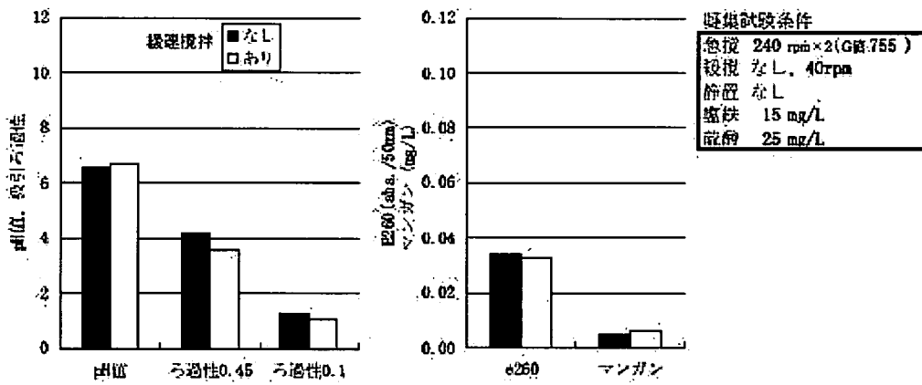
図-F-8 緩速撹拌の有無と処理水質の関係(静置なし)
