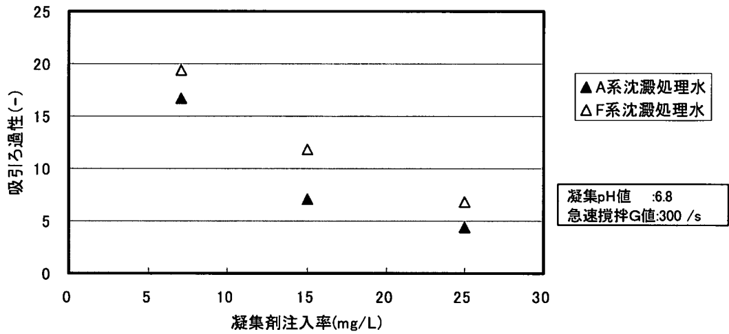
図 11 凝集剤注入率と吸引ろ過性の関係[平均値]
