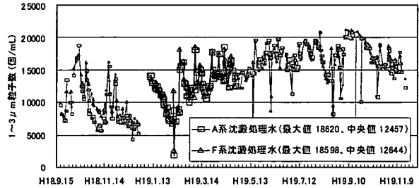
図 4-3-60 連続実験 RUN2 1~3 μm 粒子数 沈澱処理水
