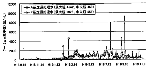
図 4-3-66 連続実験 RUN2 7~12 \mu m 粒子数 沈澱処理水
