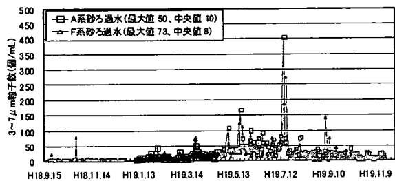
図 4-3-65 連続実験 RUN2 3~7 \mu m 粒子数 砂ろ過水
