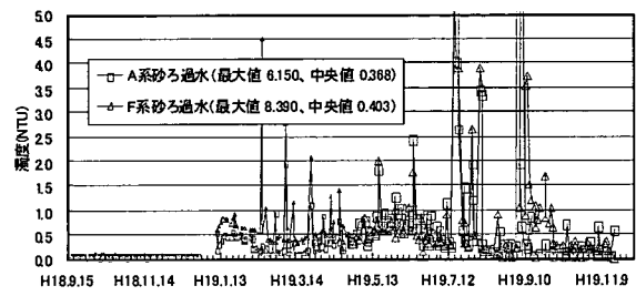
図 4-3-78 連続実験 RUN3 砂ろ過水濁度 (卓上分析)
