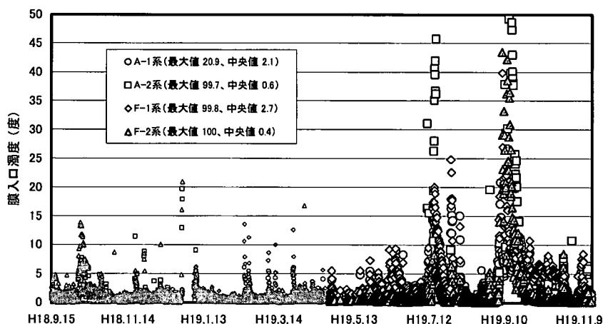
図 4-3-76 連続実験 RUN3 膜入口濁度
