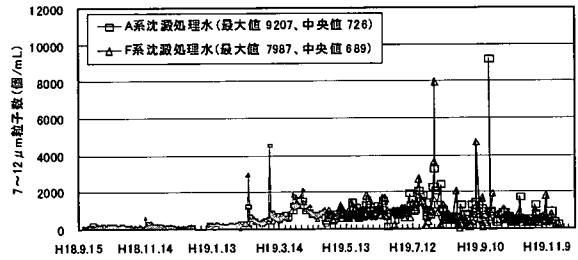
図 4-3-102 連続実験 RUN3 7~12 μm 粒子数 沈澱処理水
