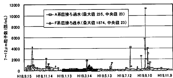
図 4-3-67 連続実験 RUN2 7~12 \mu m 粒子数 直接ろ過水
