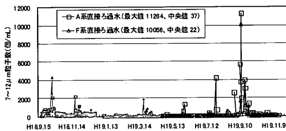
図 4-3-103 連続実験 RUN3 7~12 μm 粒子数 直接ろ過水
