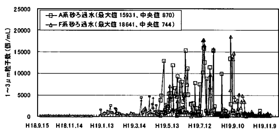
図 4-3-98 連続実験 RUN3 1\sim 3\mu\text{m} 粒子数 砂ろ過水
