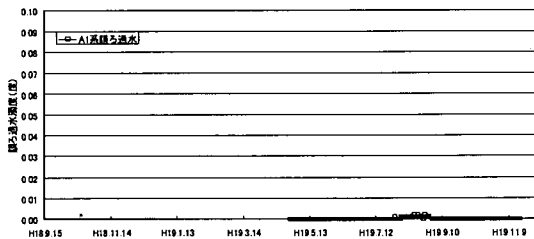
図 4-3-81 連続実験 RUN3 A-1 膜ろ過水濁度
