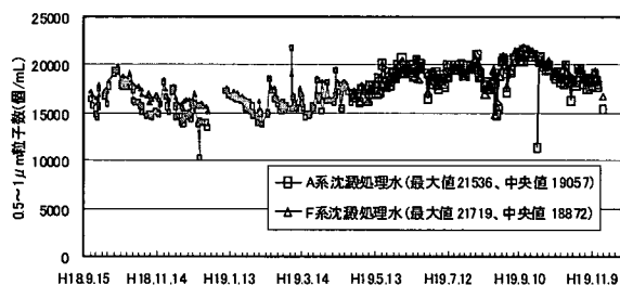
図 4-3-93 連続実験 RUN3 0.5\sim 1\mu\text{m} 粒子数 沈澱処理水
