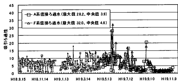
図 4-3-92 連続実験 RUN3 吸引ろ過性
