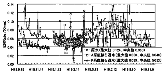
図 4-3-52 連続実験 RUN2 E260
