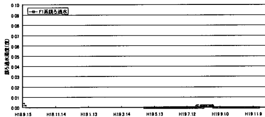
図 4-3-79 連続実験 RUN3 F-1 膜ろ過水濁度
