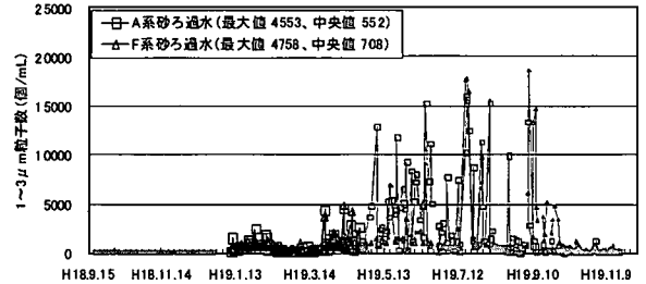
図 4-3-62 連続実験 RUN2 1~3 μm 粒子数 砂ろ過水
