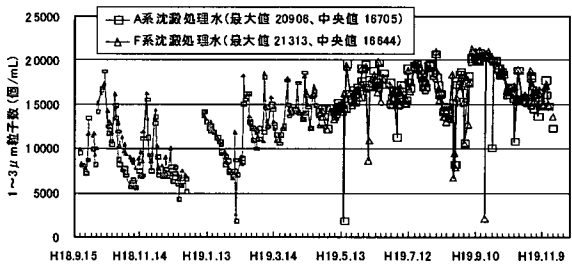
図 4-3-96 連続実験 RUN3 1\sim 3\mu\text{m} 粒子数 沈澱処理水
