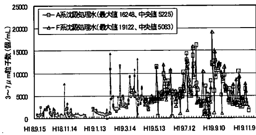
図 4-3-99 連続実験 RUN3 3~7 μm 粒子数 沈澱処理水
