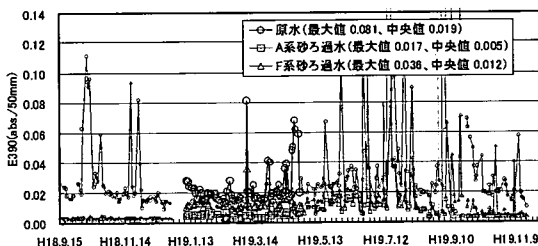
図 4-3-49 連続実験 RUN2 色度 原水・砂ろ過水
