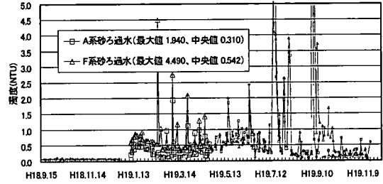
図 4-3-46 連続実験 RUN2 砂ろ過水濁度 (卓上分析)
