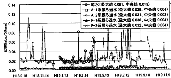
図 4-3-50 連続実験 RUN2 色度 原水・膜ろ過水
