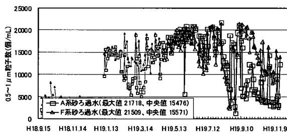
図 4-3-95 連続実験 RUN3 0.5\sim 1\mu\text{m} 粒子数 砂ろ過水
