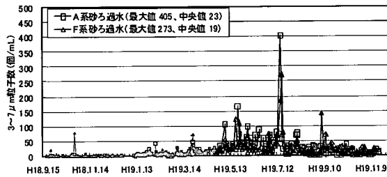
図 4-3-101 連続実験 RUN3 3~7 μm 粒子数 砂ろ過水
