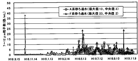
図 4-3-104 連続実験 RUN3 7~12 μm 粒子数 砂ろ過水
