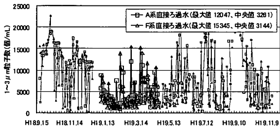
図 4-3-61 連続実験 RUN2 1~3 μm 粒子数 直接ろ過水
