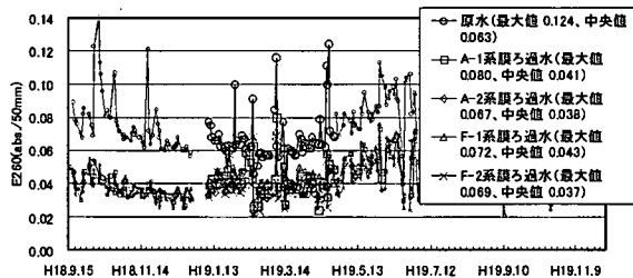
図 4-3-54 連続実験 RUN2 E260
