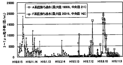
図 4-3-100 連続実験 RUN3 3~7 μm 粒子数 直接ろ過水
