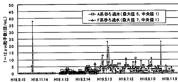
図 4-3-68 連続実験 RUN2 7~12 \mu m 粒子数 砂ろ過水
