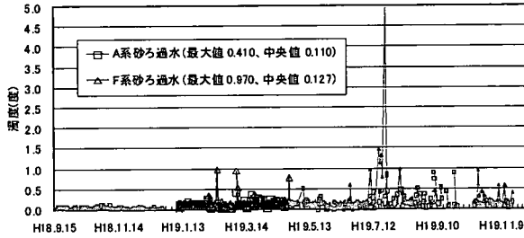
図 4-3-45 連続実験 RUN2 砂ろ過水濁度 (自動計測)
