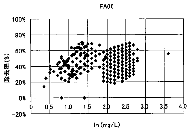
図 3-3-219 入口 TOC と除去率の関係
