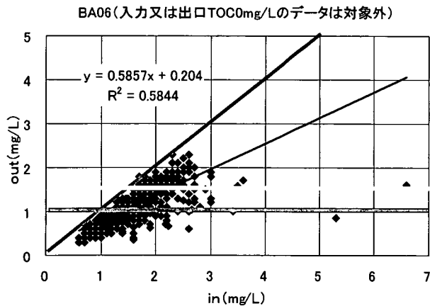
図 3-3-204 入口 TOC と出口 TOC の関係
