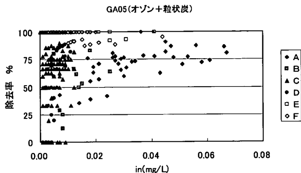
図 3-3-197 入口マンガンと除去率の関係-2
