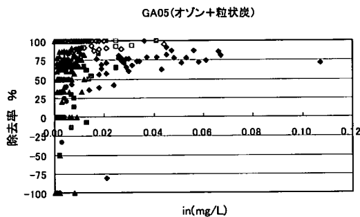
図 3-3-196 入口マンガンと除去率の関係-1
