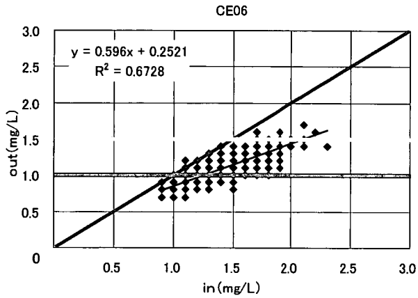
図 3-3-214 入口 TOC と出口 TOC の関係
