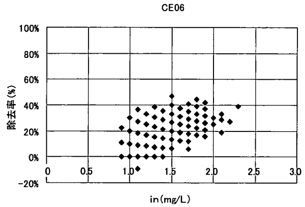
図 3-3-215 入口 TOC と除去率の関係
