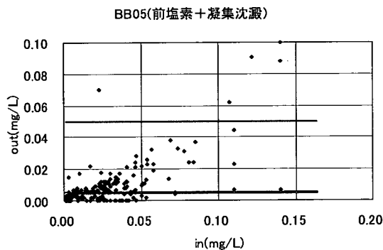
図 3-3-186 入口マンガンと出口マンガンの関係
