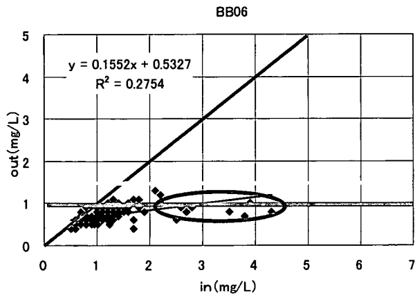
図 3-3-206 入口 TOC と出口 TOC の関係
