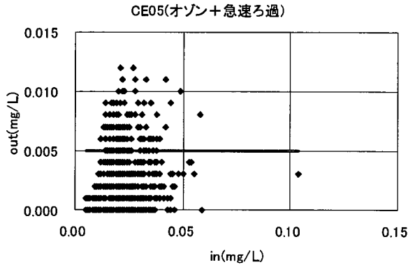
図 3-3-192 入口マンガンと出口マンガンの関係
