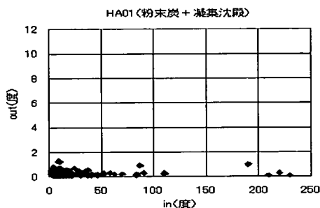
図 3-3-153 入口濁度と出口濁度の関係
