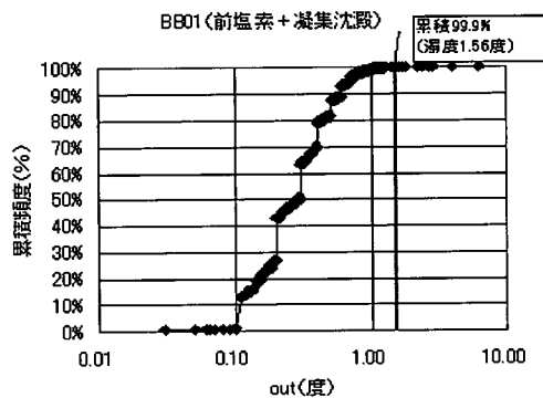
図 3-3-140 出口濁度の累積頻度
