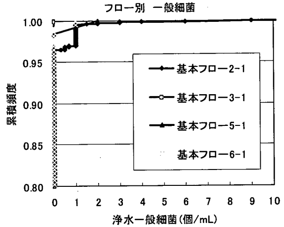
図 3-3-125 浄水の累積頻度
