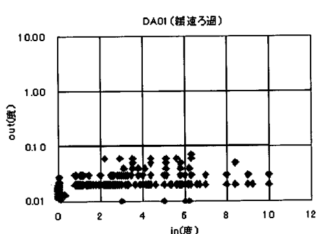
図 3-3-149 入口濁度と出口濁度の関係
