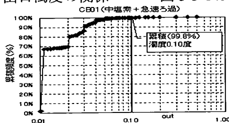
図 3-3-146 出口濁度の累積頻度
