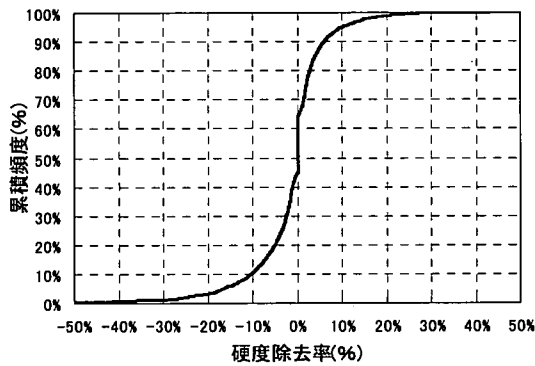
図 3-3-133 硬度除去率の累積頻度
