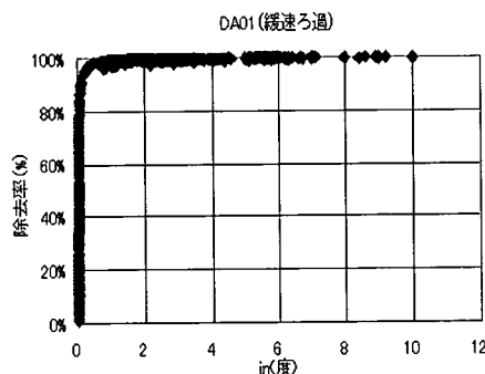
図 3-3-150 入口濁度と除去率の関係
