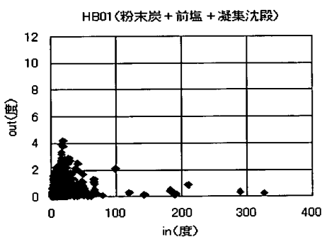
図 3-3-155 入口濁度と出口濁度の関係
