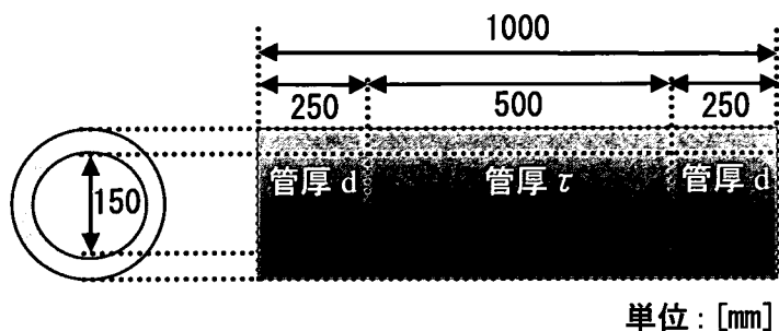
図 5. 5. 19 解析モデル詳細
