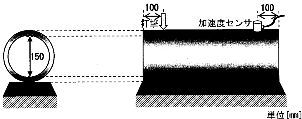
図 5.5.6 供試管の設置状況および弾性波計測方法
