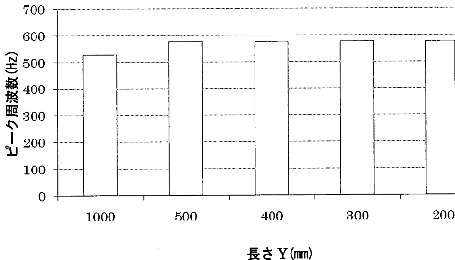
図 5. 5. 24 部分的な減肉の長さとのピーク周波数の関係
