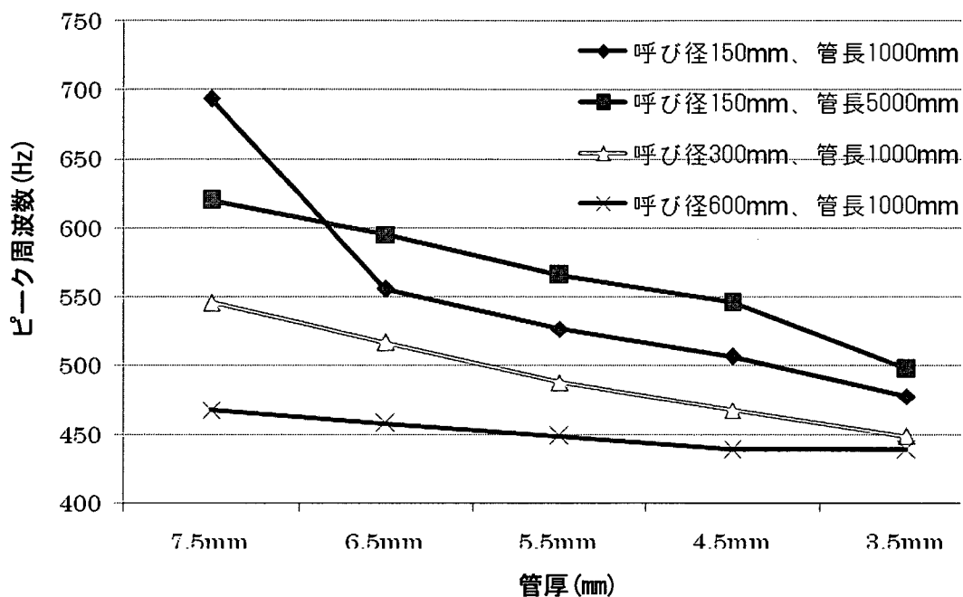
図 5.5.14 管径および管長の異なる管ごとの管長とピーク周波数の関係
