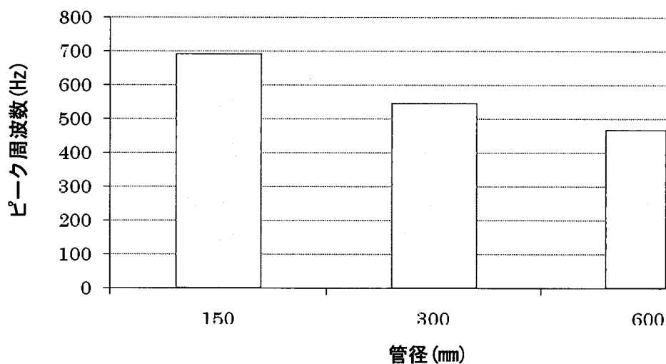
図 5.5.13 管径とピーク周波数の関係
