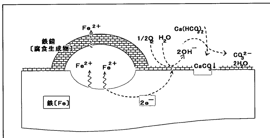
図 3.6.28 鉄の腐食による炭酸カルシウム析出モデル
