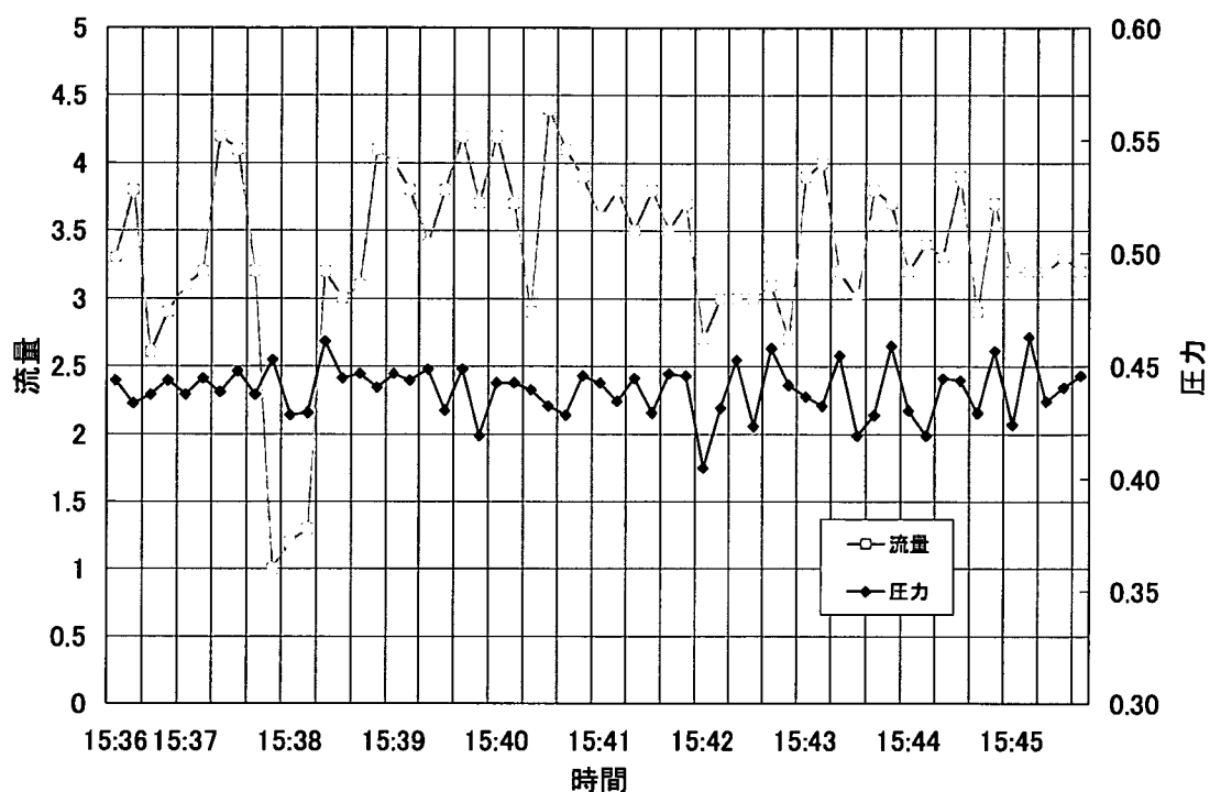
図 3. 6. 20 ランゲリ指数未改善側の管内観察時の流量と圧力 (0 保育所)
