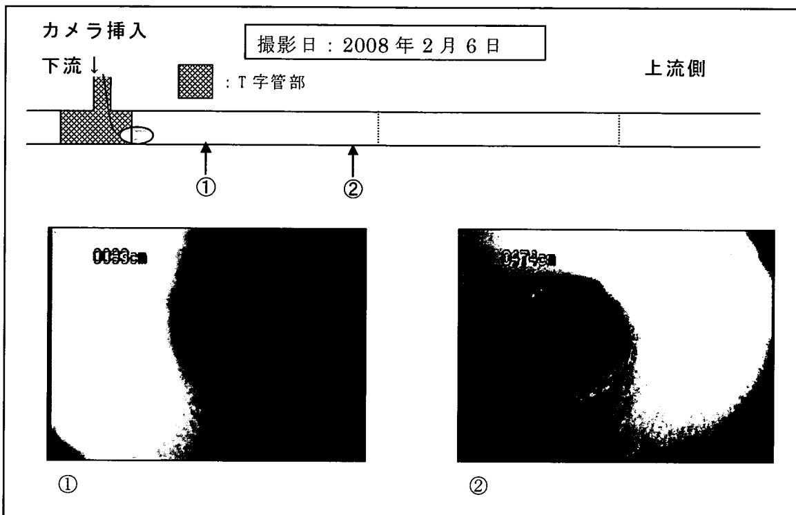
写真 3. 6. 16 ランゲリア指数未改善側での上流側管内状態（〇保育所）
