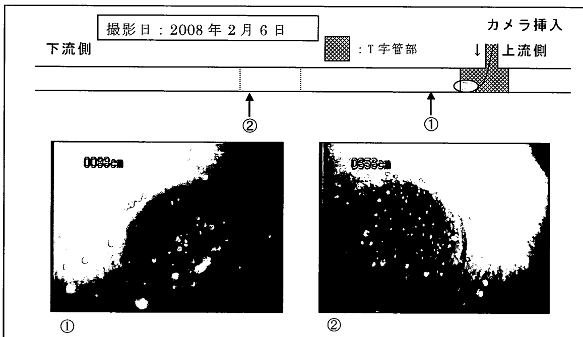
写真 3. 6. 17 ランゲリア指数未改善側での下流側管内状態（〇保育所）
