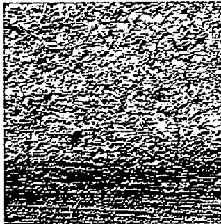
BSE像
