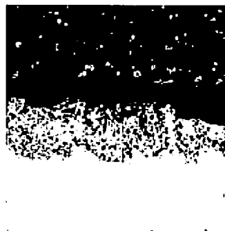
Ca
