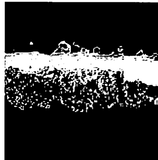
Si
