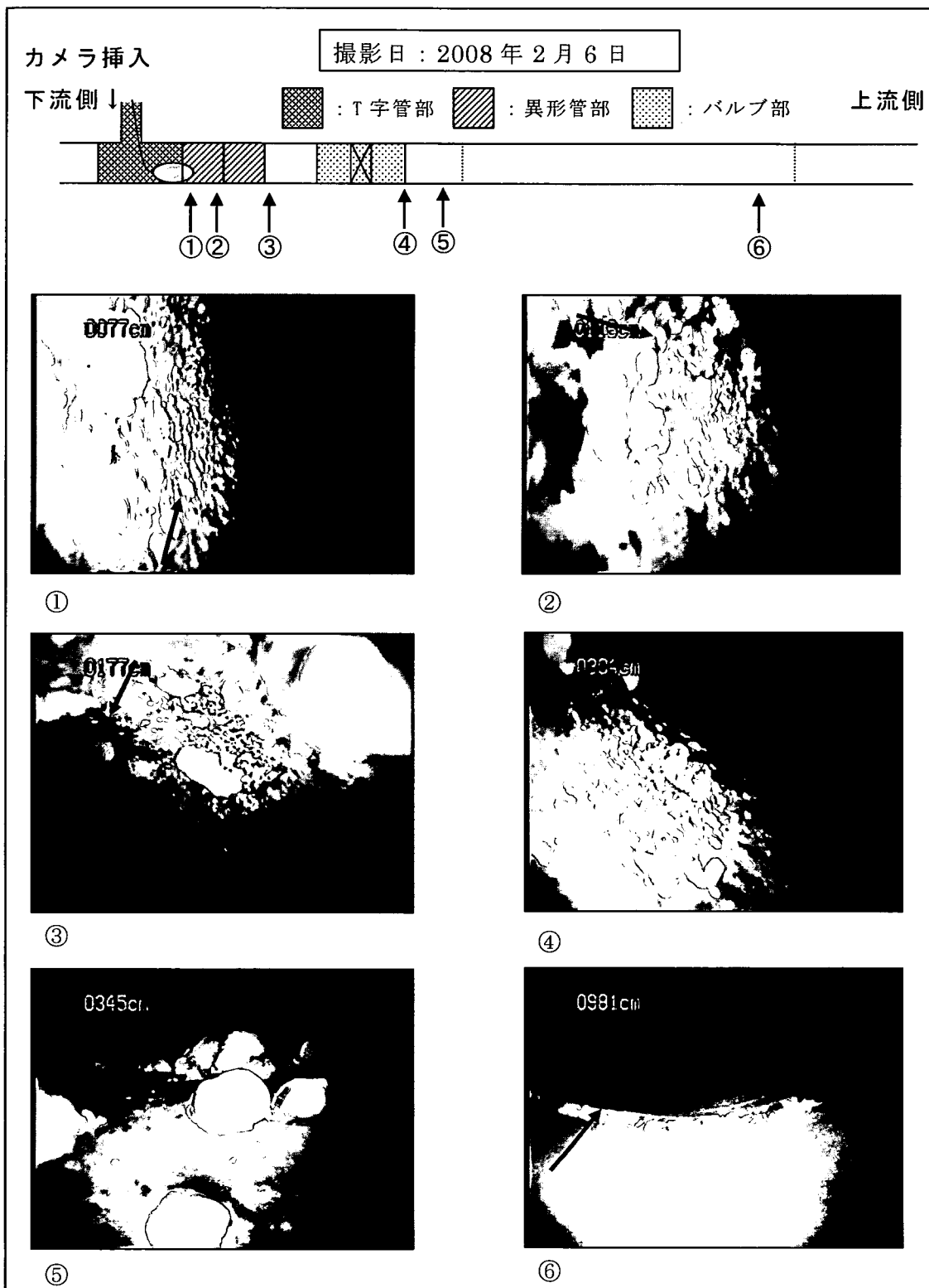
写真 3. 6. 14 ランゲリア指数未改善側での上流側管内状態 (N運動場)
