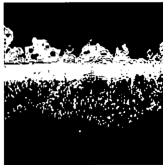
Si
