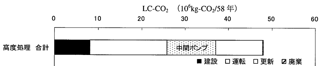
図 3-5-14 「凝集沈澱+オゾン+活性炭+砂ろ過」のフロー全体の LC-CO 2
