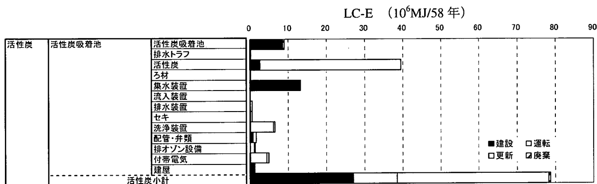
図 3-5-11 活性炭吸着池のライフサイクルエネルギー消費量 (LC-E) 算出結果 (設備毎の累積)
