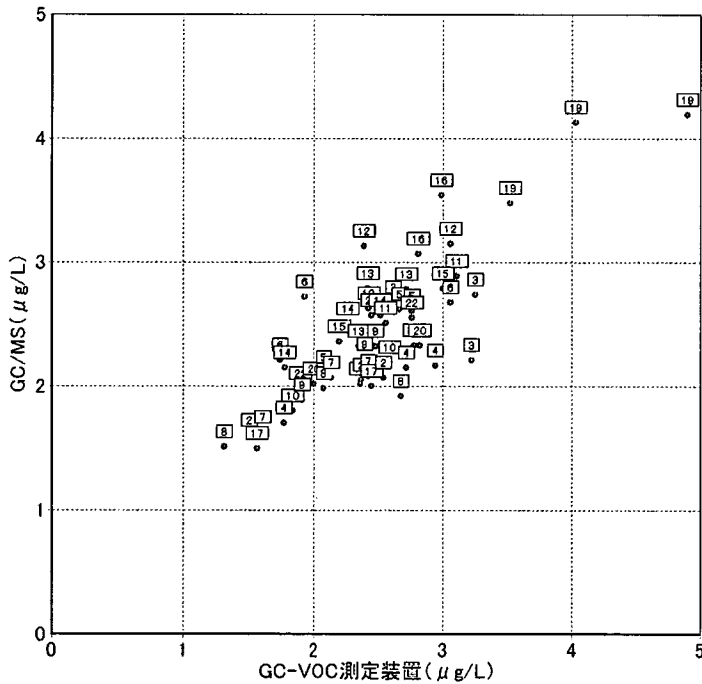
図6 VOC測定装置とGC/MS測定値の相関 2.5 \mu g/L希釈液の場合
