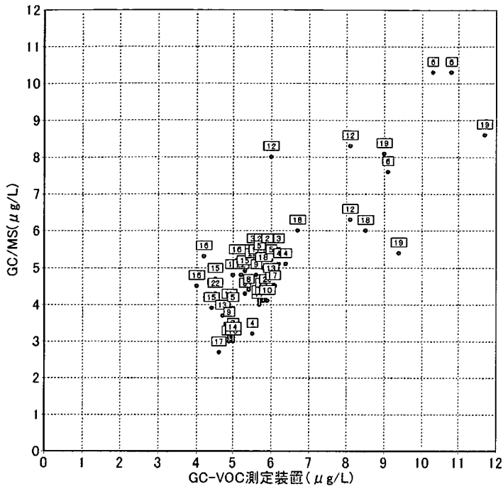
図5 VOC測定装置とGC/MS測定値の相関 5 \mu g/L希釈液の場合
