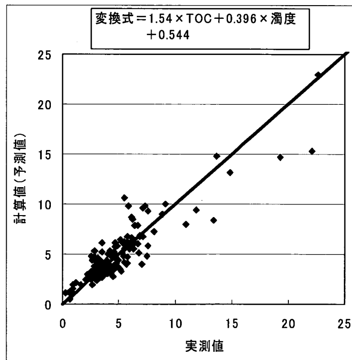
図 過マンガン酸カリウム消費量 実測値と予測値の関係
