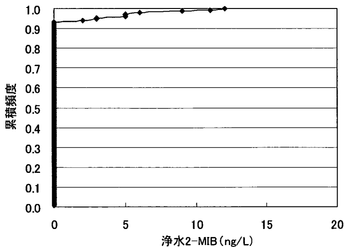
図 3-3-98 基本フロー5-1+6-1 (高度処理) の原水中 2-MIB の存在割合
