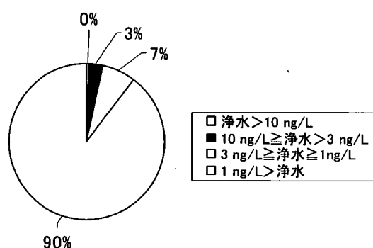
図 3-3-93 基本フロー2-1b (粉末炭あり) の浄水中 2-MIB 濃度の存在割合
