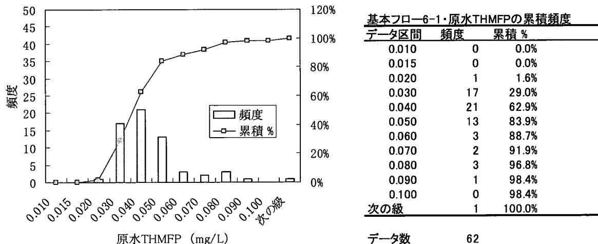
図 3-3-121 基本フロー6-1 原水 THMFP の累積頻度
