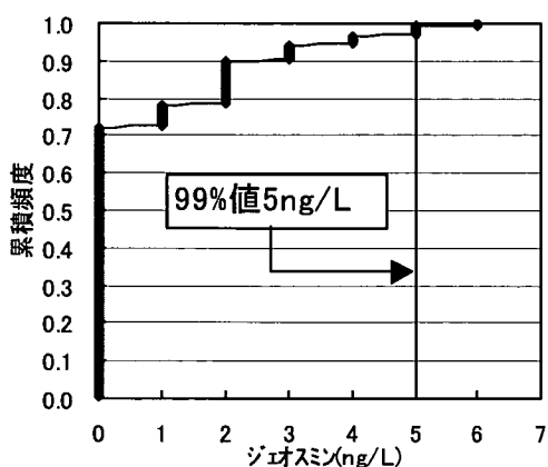
図 3-3-103 フロー2-1a の原水の累積頻度
