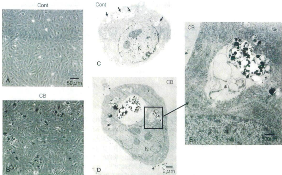
図 1. カーボンブラック (CB) 処置後, 血管内皮細胞の光学および電子顕微鏡像 A: 正常内皮細胞 (光学顕微鏡レベル), B: CB 処置後内皮細胞 (光学顕微鏡レベル), C: 正常内皮細胞 (電子顕微鏡レベル), D: CB 処置後内皮細胞 (電子顕微鏡レベル), E: CB の食胞への取り込み, 矢印: 食胞, *: 拡張した食胞, N: 核. (Yamawaki H et al , 2006 3) より改変引用)
