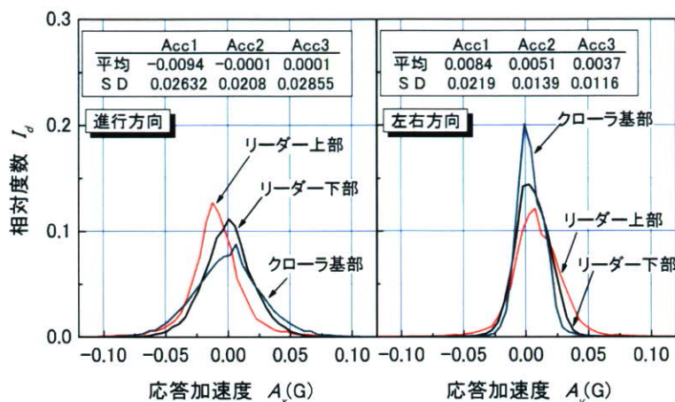
図 3-7-20 応答加速度の相対度数の分布
