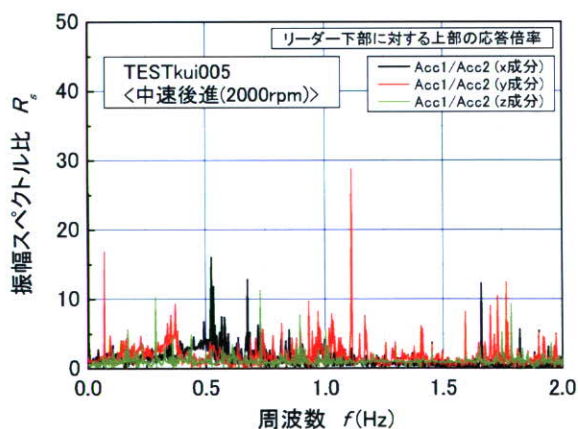
図 3-7-24 リーダー下部に対する上部の応答倍率 x, y, z 方向の 3 成分 (TESTkui005)
