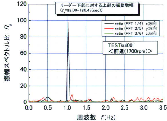
図 3-7-10 リーダー下部に対する上部の応答倍率比 (x, y, z 方向の 3 成分)
