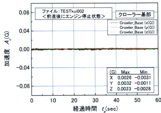
c) クローラ基部における応答
