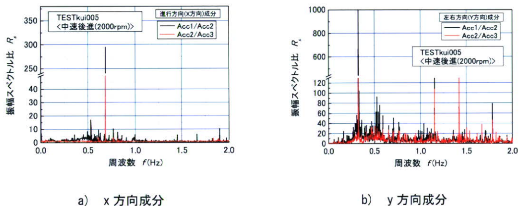
図 3-7-23 クローラ基部に対するリーダー下部と上部における加速度振幅の応答比較 (TESTkui005)
