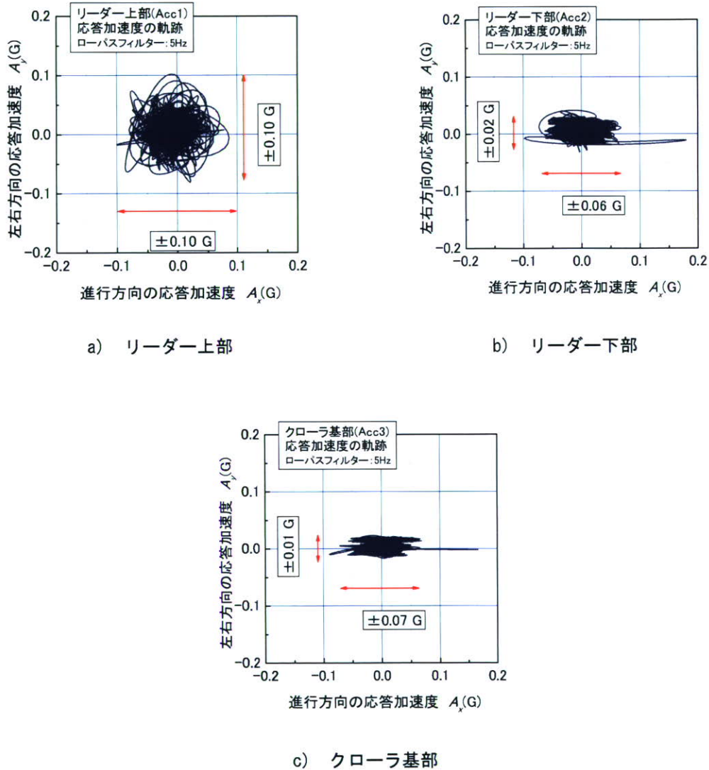
図 3-7-19 応答加速度の平面軌跡
