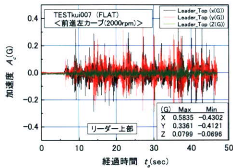
a) リーダー上部における応答
