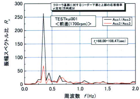
b) y 方向成分
