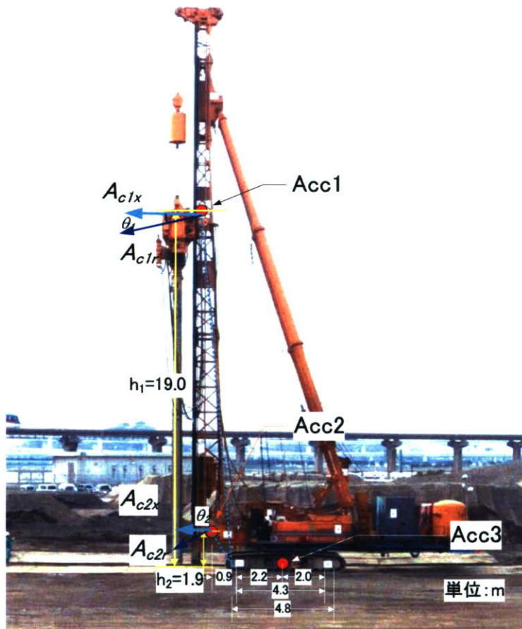
写真 3-7-1 前輪を中心とした回転による応答加速度
