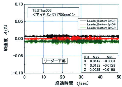
b) リーダー下部における応答
