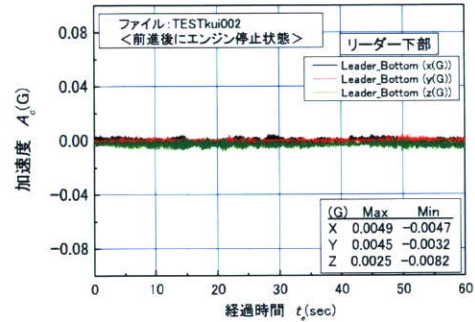
b) リーダー下部における応答
