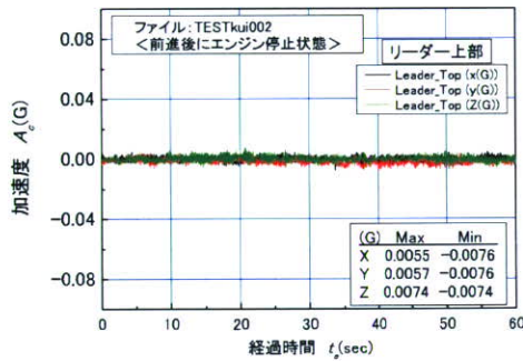
a) リーダー上部における応答
