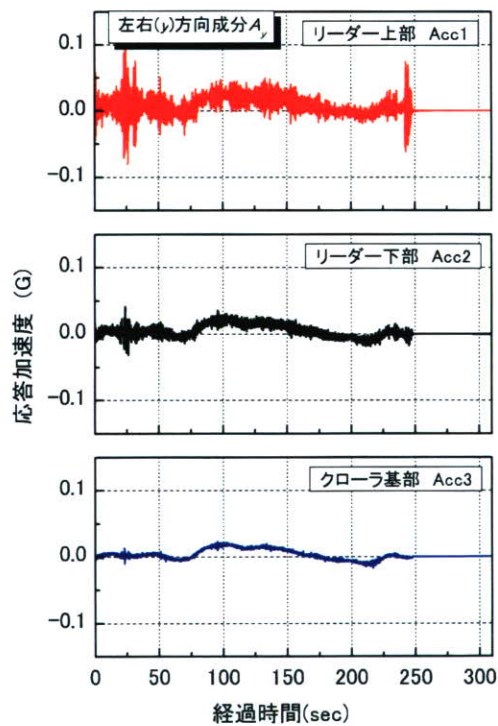
b) 左右(y)方向成分
