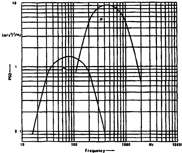
図3 新 JIS T 8114で使用する振動スペクトル
