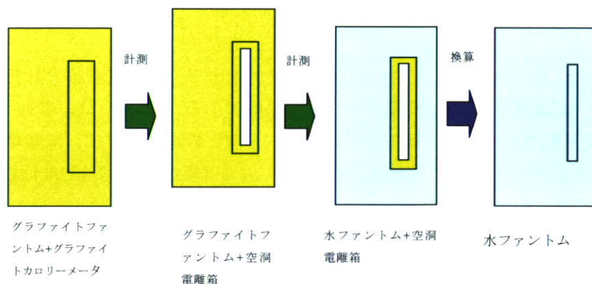
図7 グラファイトカロリメータから水吸収線量評価のためのステップ概念図
