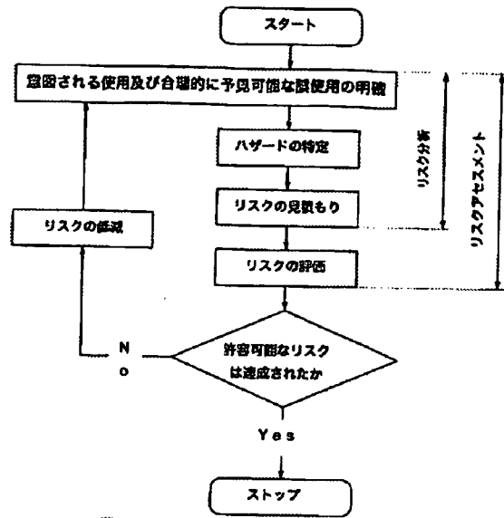
図1 リスクアセスメントおよびリスク低減の反復プロセス
